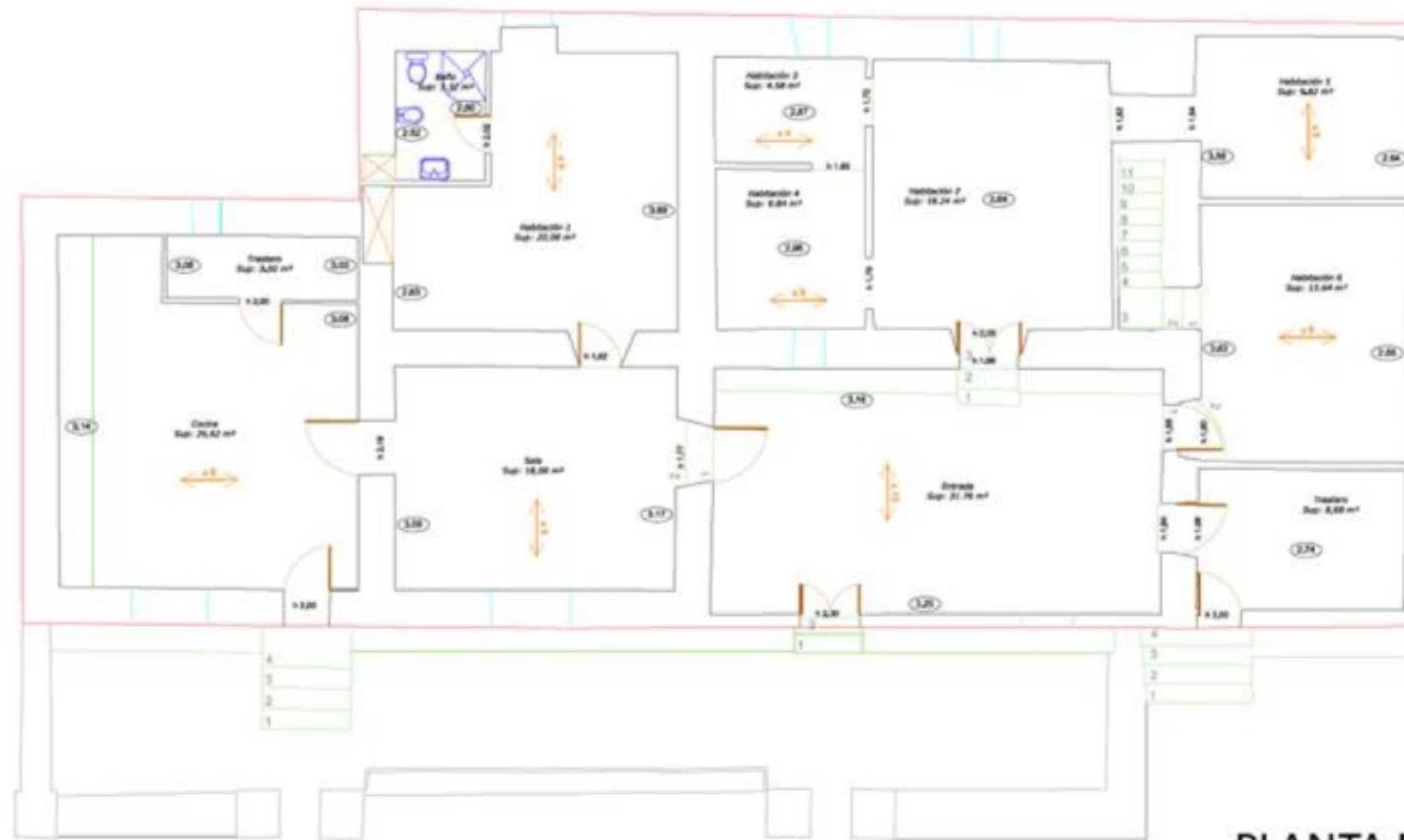
PLANTA BAJA
