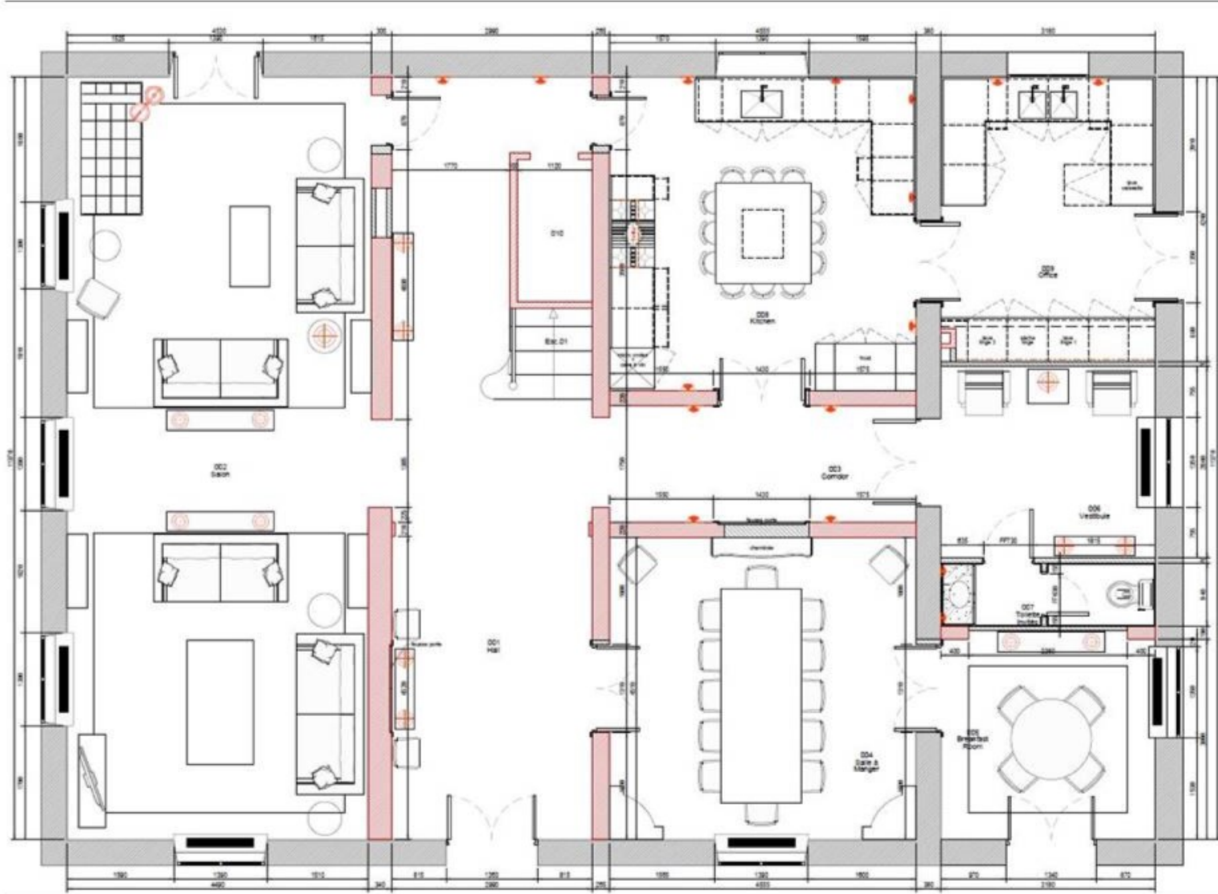
CASA PRINCIPAL, PLANTA BAJA
