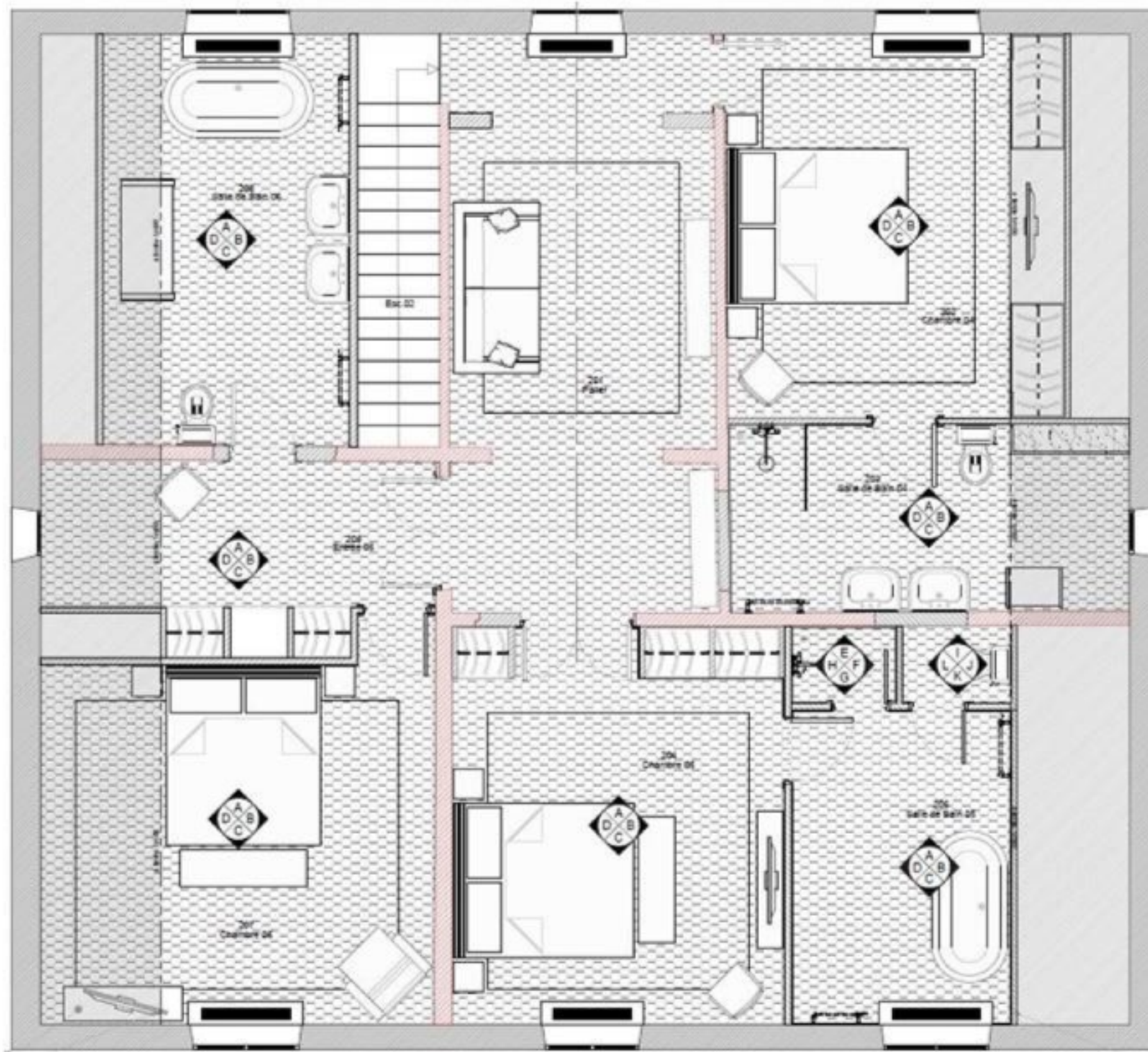
CASA PRINCIPAL, PLANTA SEGUNDA
