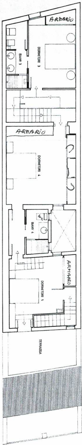
PLANTA PIS
