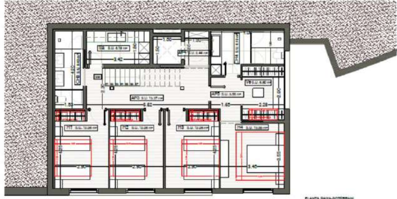
PLANTA SÓTANO
