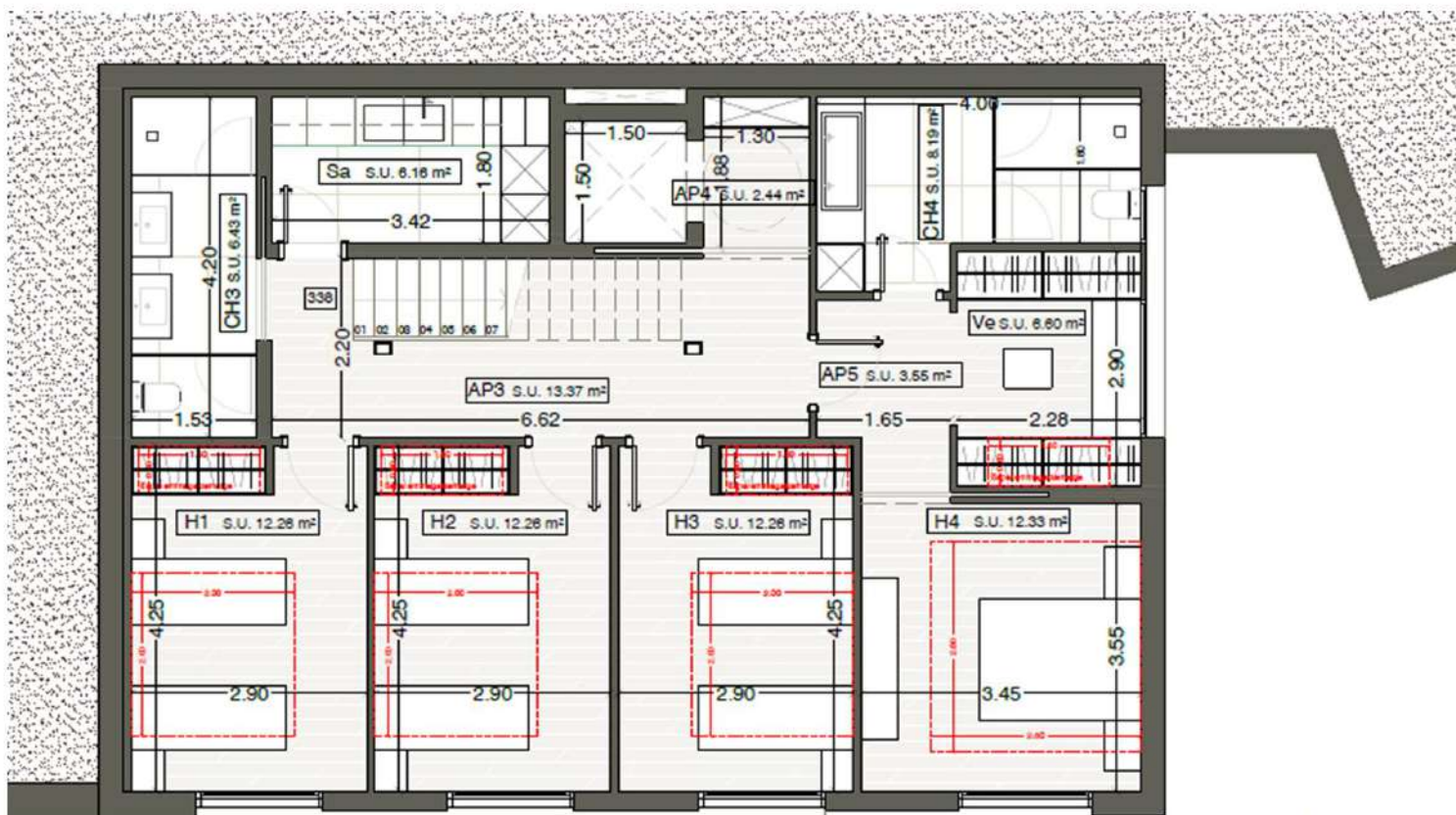
PLANTA BAIXA-SOTERRANI
