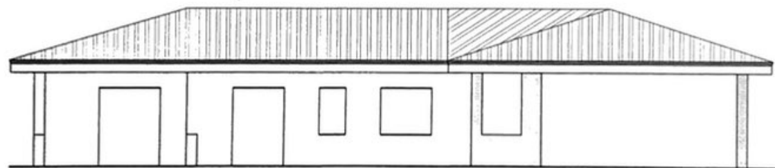
ALÇAT SUD
