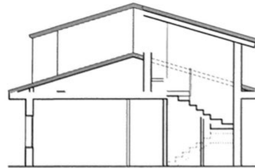
SECCIÓ C
