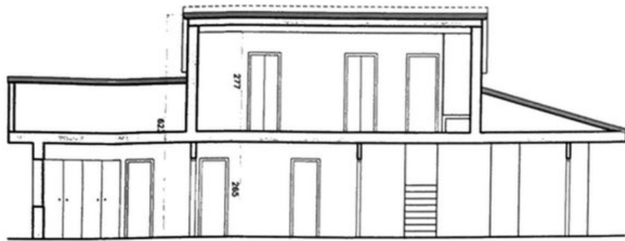
SECCIÓ A
