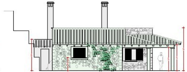
Alzado lateral izquierdo
