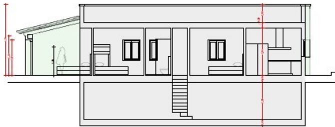
Seccion longitudinal
