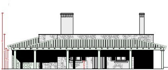
Alzado Frontal
