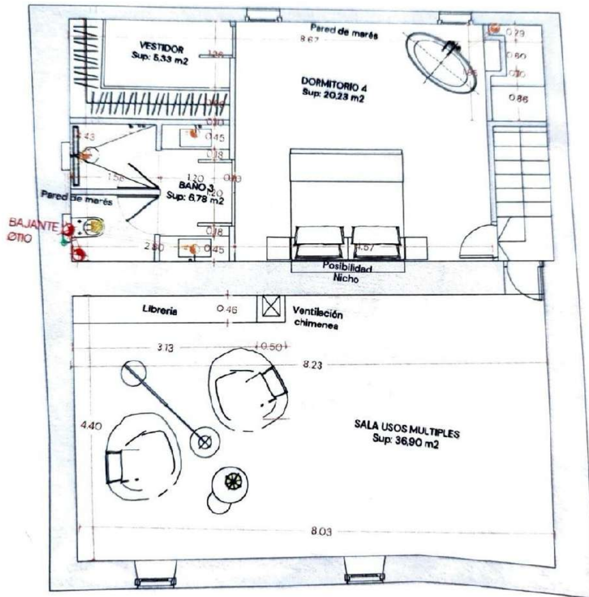
PLANTA SEGUNDA
