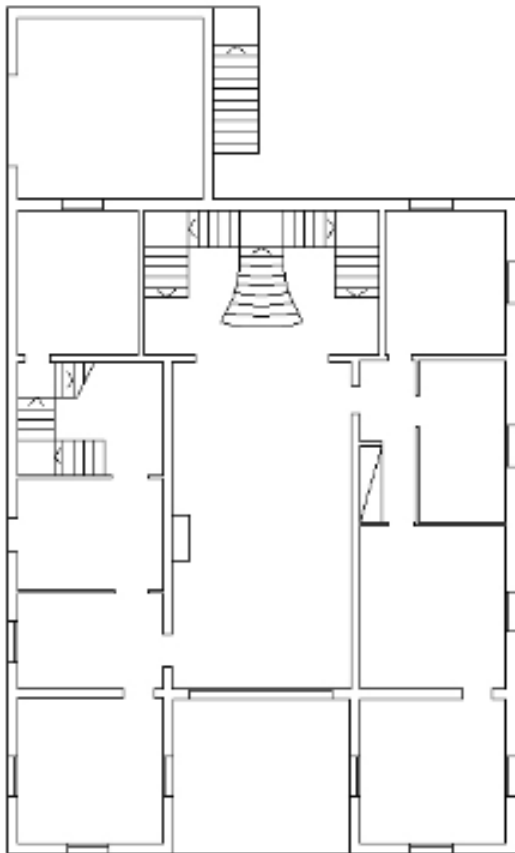
PLANTA BAJA
