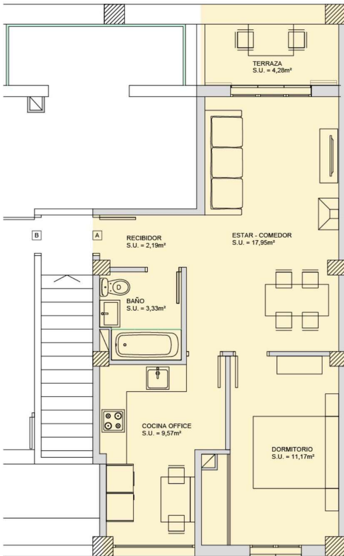
PLANTA APARTAMENTO PISO A SUPERFICIE ÚTIL APARTAMENTO = 48,49m² SUPERFICIE TOTAL CONSTRUIDA = 57,18m² E.1/50
