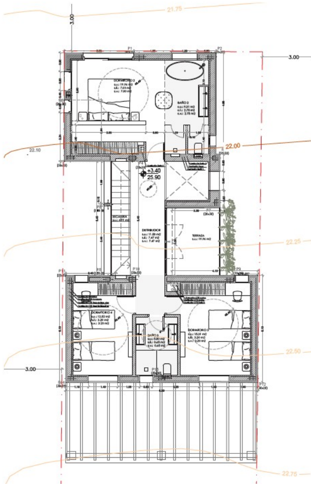
- Planta Primera 117.08 m2
