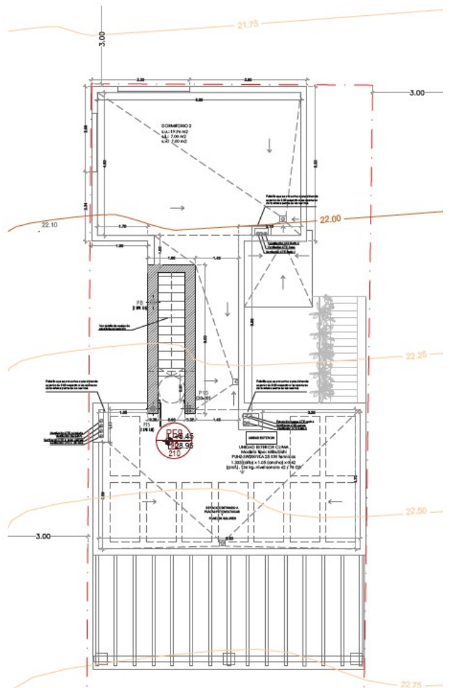
- Planta Cubierta
