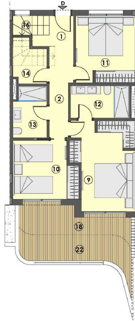
PLANTA SEGUNDA
