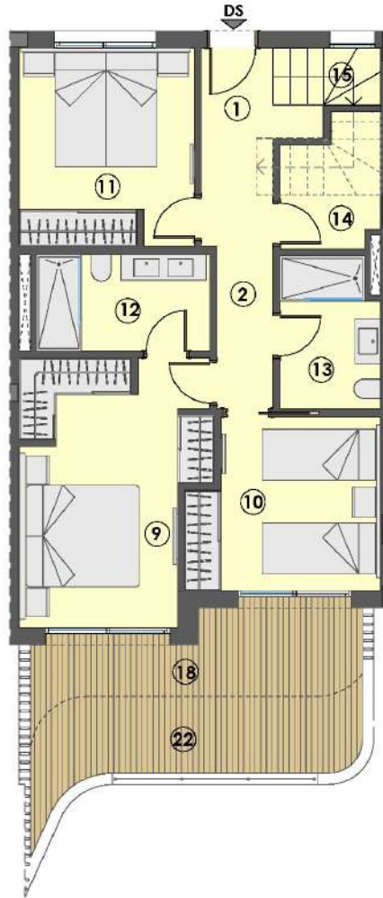
PLANTA SEGUNDA
