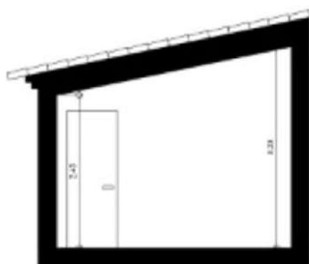
SECÇÃO C-C
