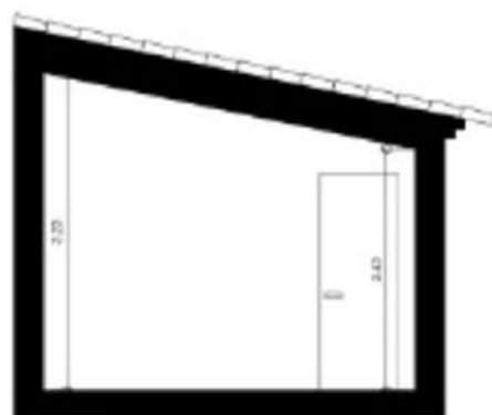
SECÇÃO A-A
