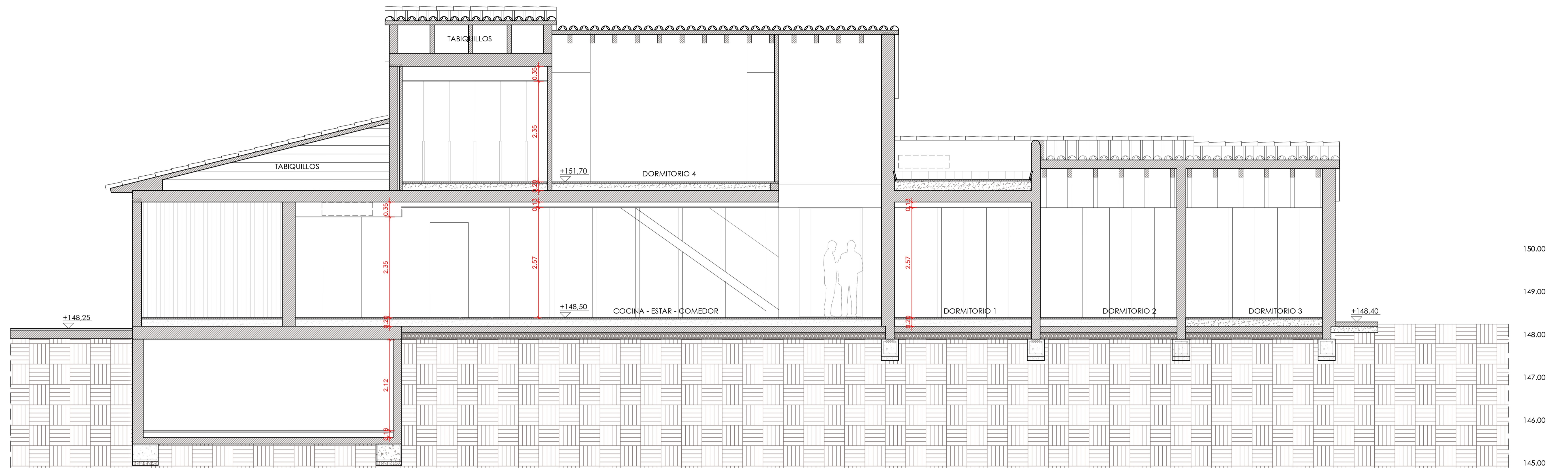
SECCIÓN A
