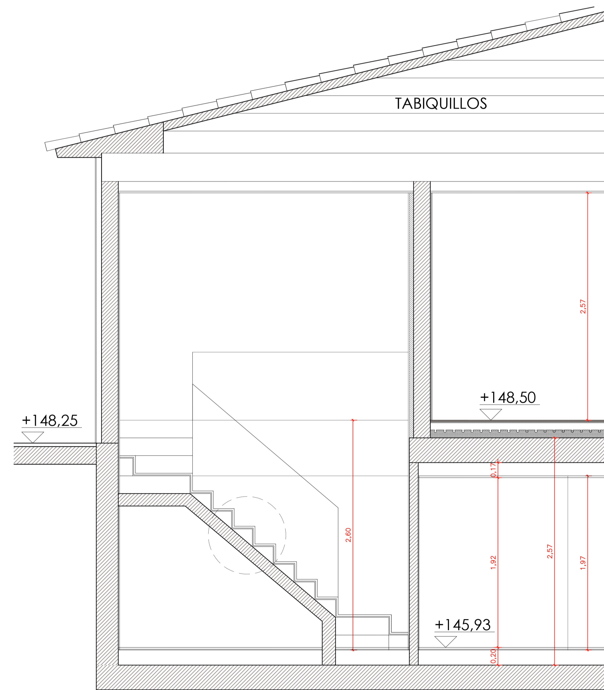
SECCION C-C'
