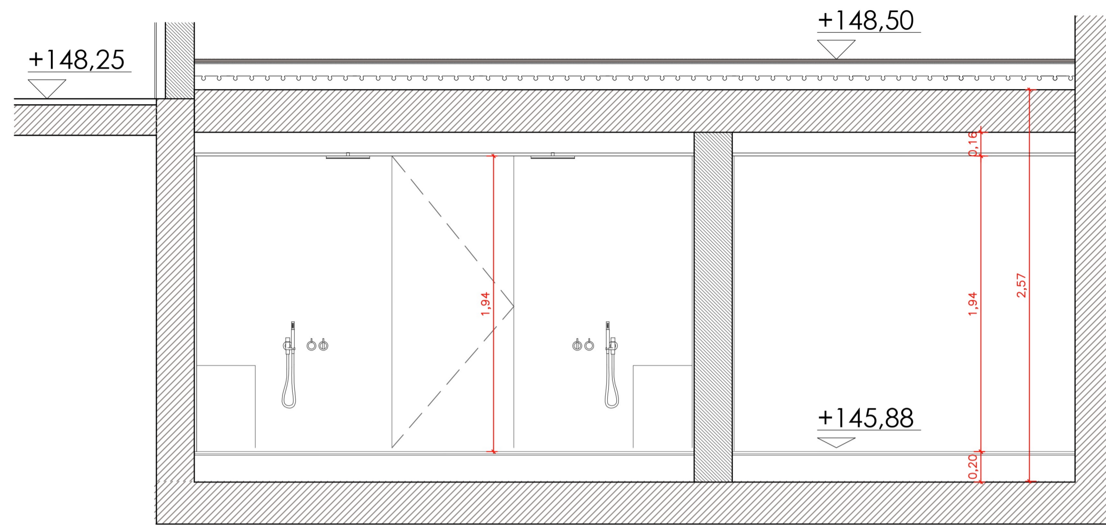
SECCION A-A'
