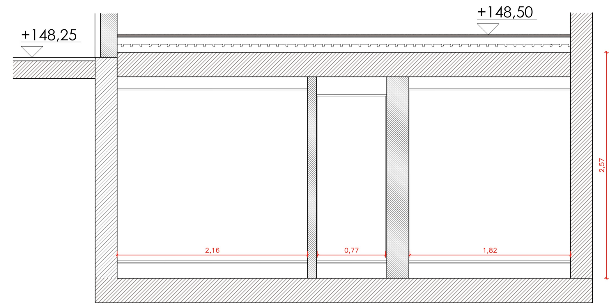
SECCION B-B'
