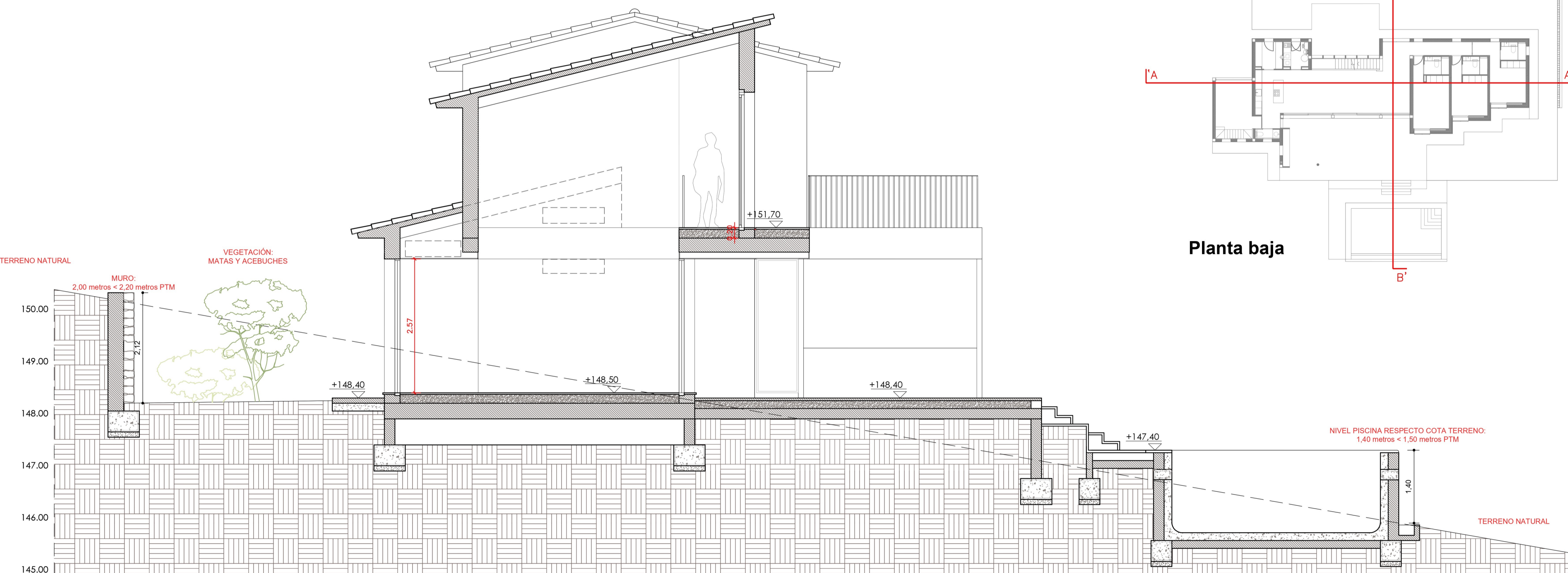
SECCIÓN B
