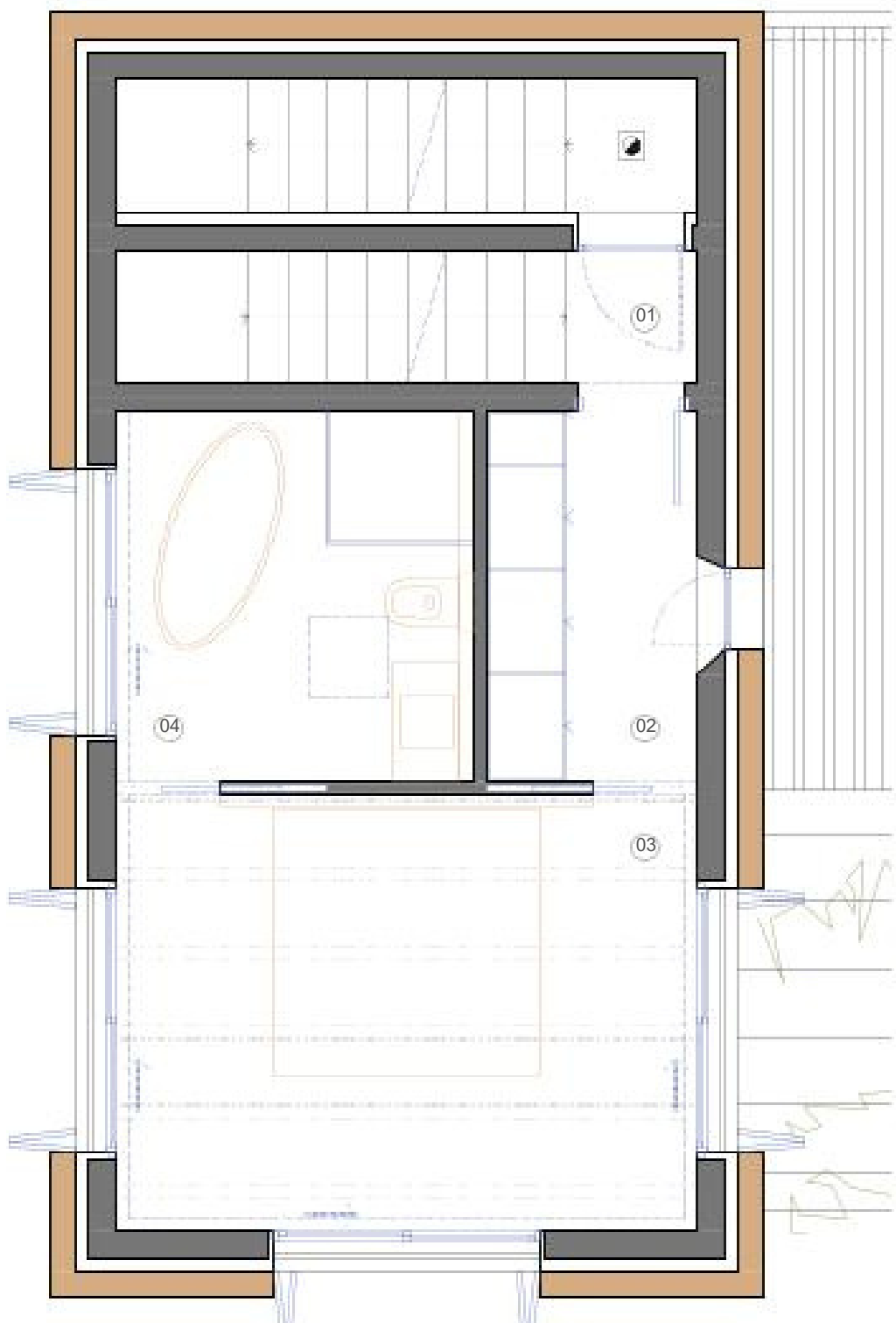
PLANTA PIS 1 · E: 1/50
