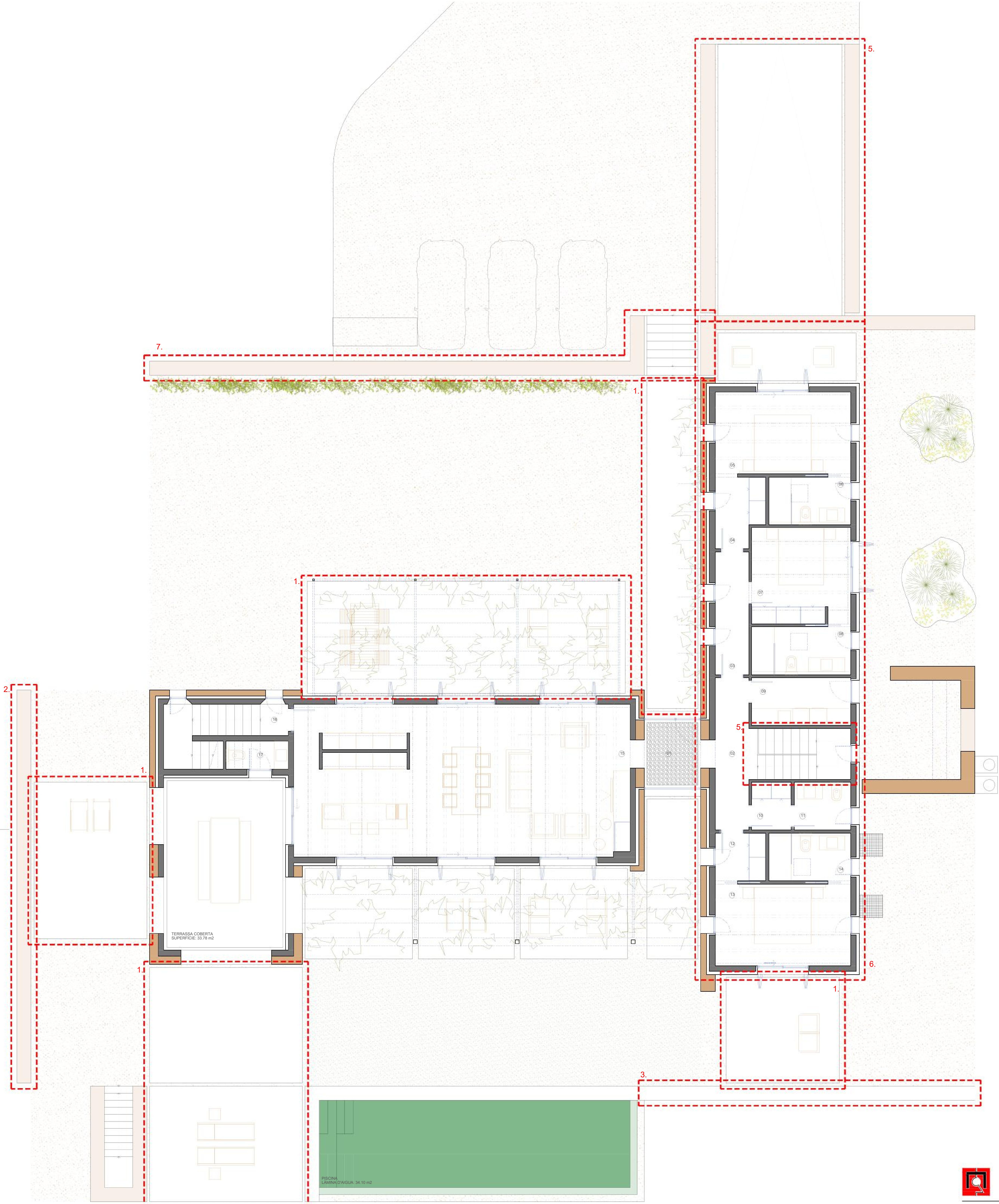
PLANTA BAIXA · E: 1/50
