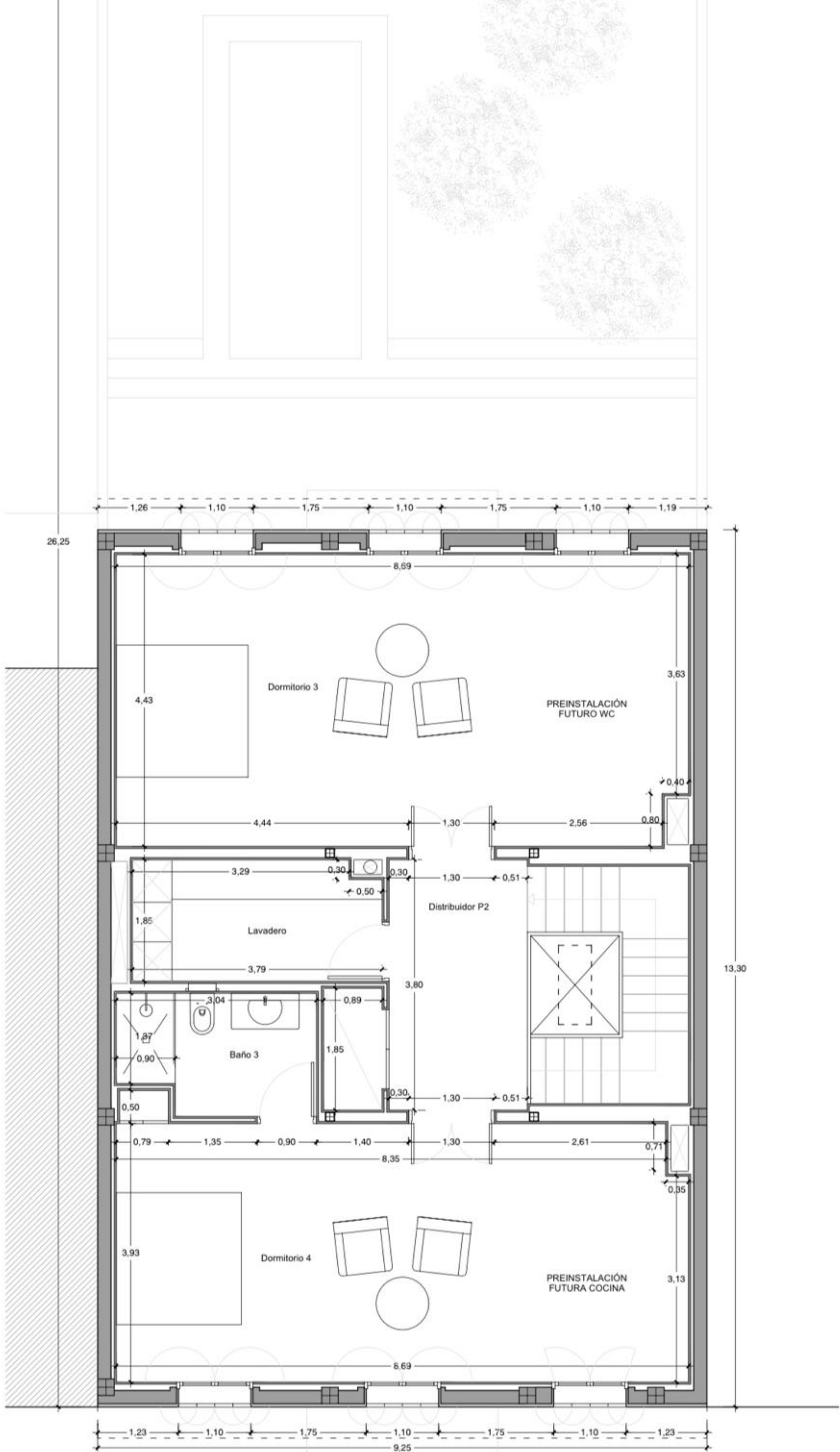
PLANTA SEGUNDA
