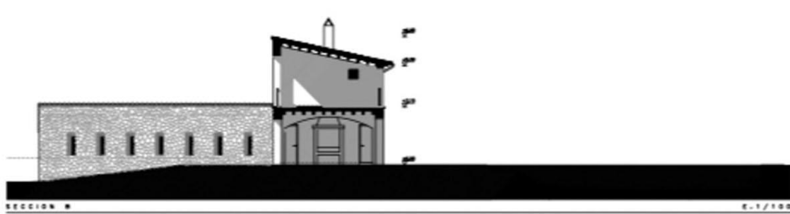
SECCION B
