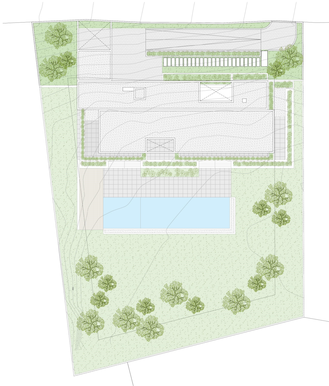
VILLA 02 SITE PLAN
