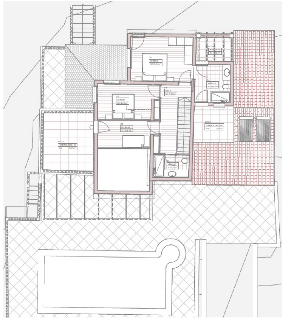
Planta Pico ESTADO MODIFICADO 150
