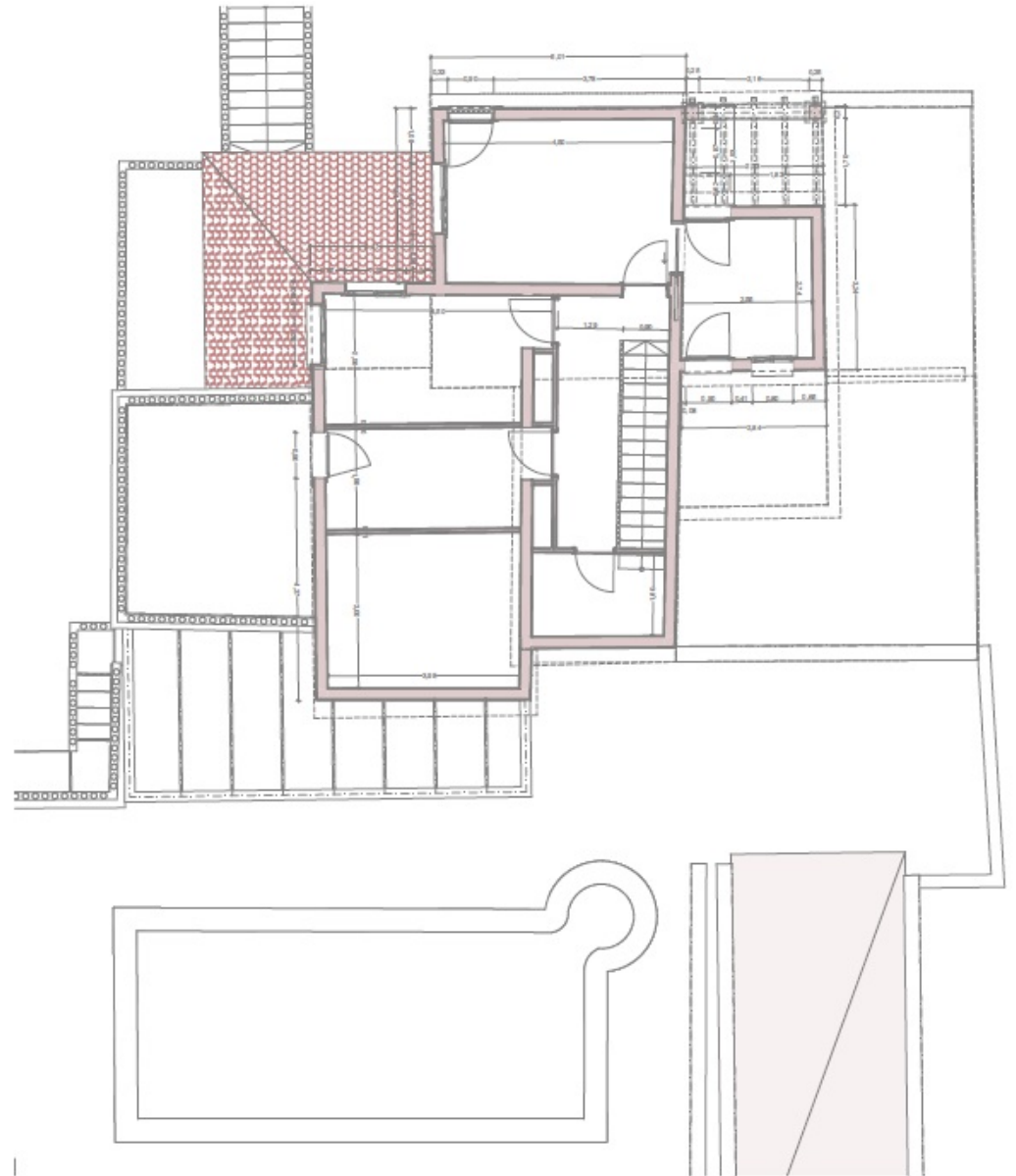
Planta Piso ESTADO MODIFICADO COTAS 150
