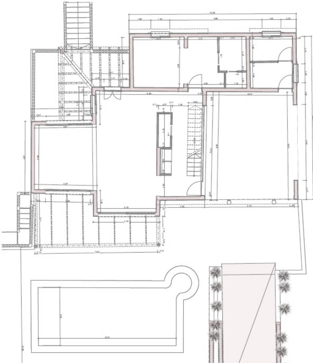
Planta Baja ESTADO MODIFICADO COTAS 150
