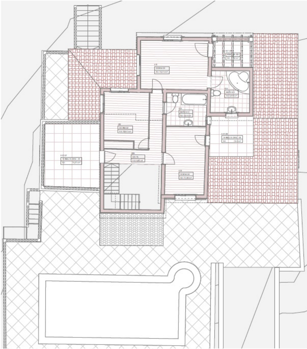
Planta Pico ESTADO ACTUAL 150
