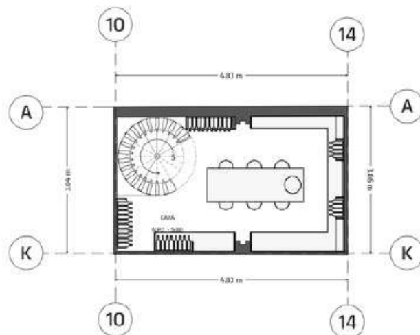
P-2 ESC 1:75
