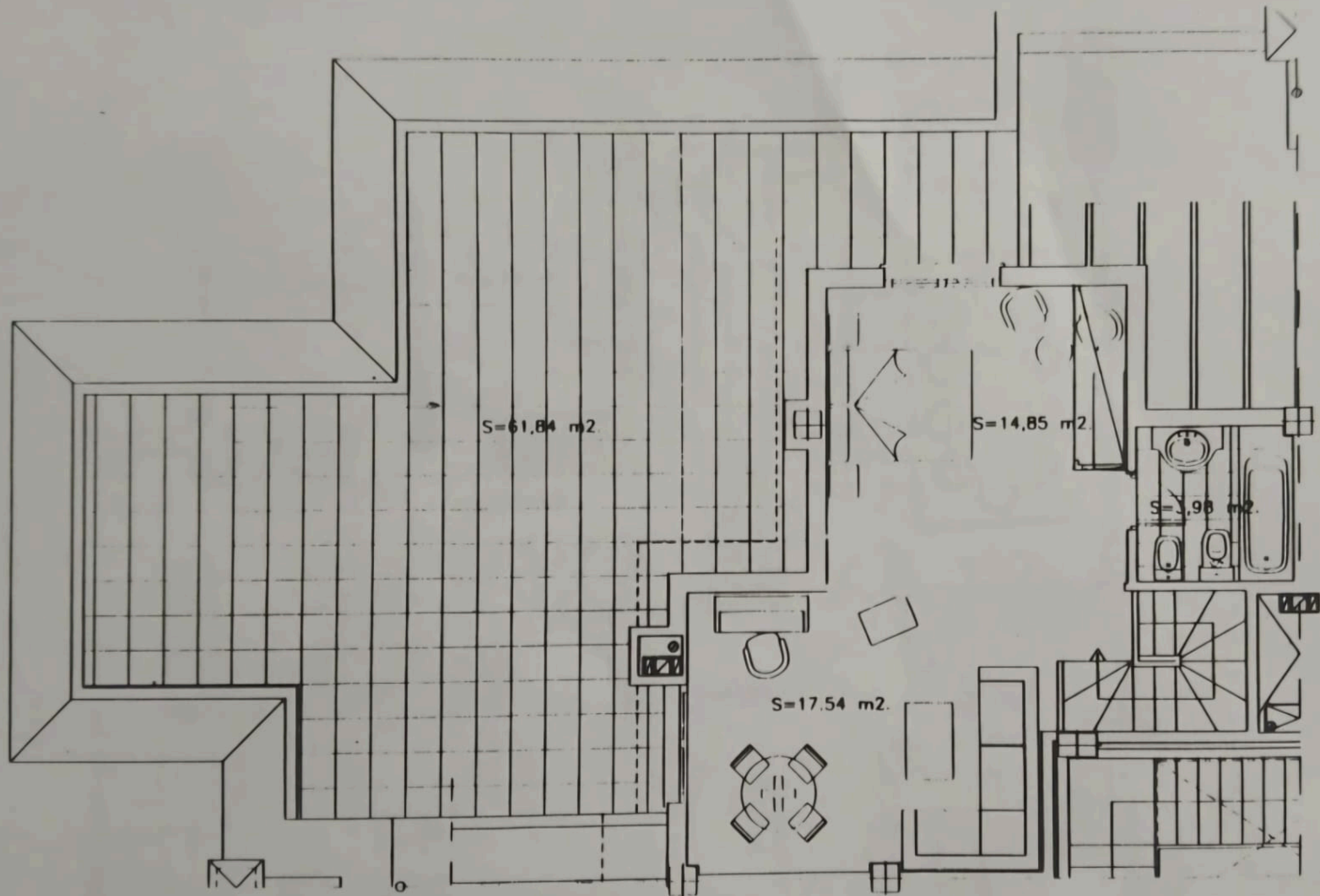
PLANTA ALTA DUPLEX PORTALES 2, 3 Y 5 VIVIENDA TIPO "D"
