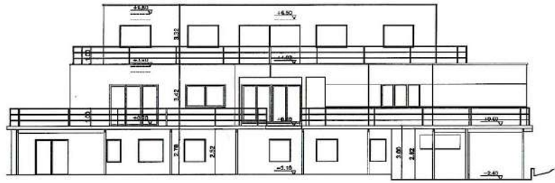
ALZADO SUR
