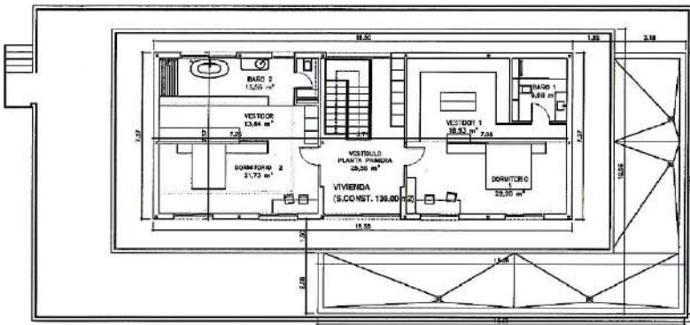
PLANTA PRIMERA
