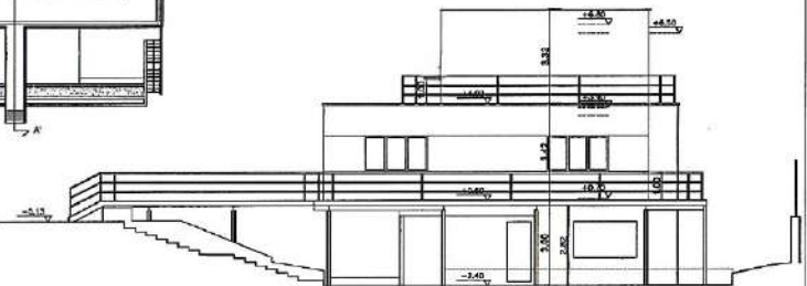
ALZADO ESTE
