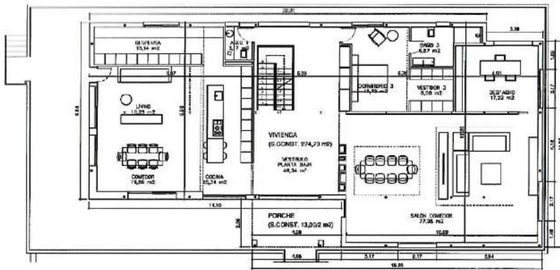
PLANTA BAJA
