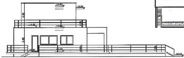
ALZADO OESTE
