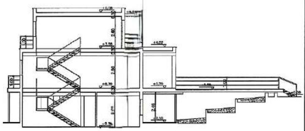
SECCION A-A'
