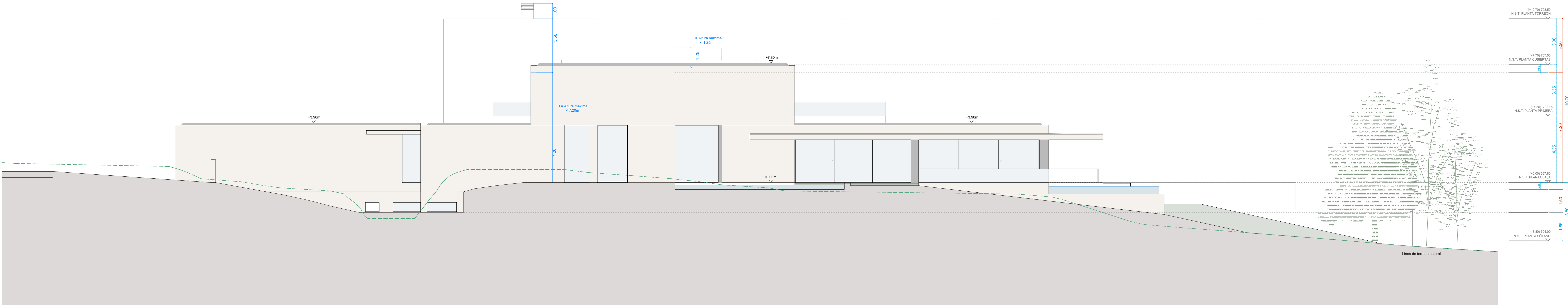
ALZADO OESTE
