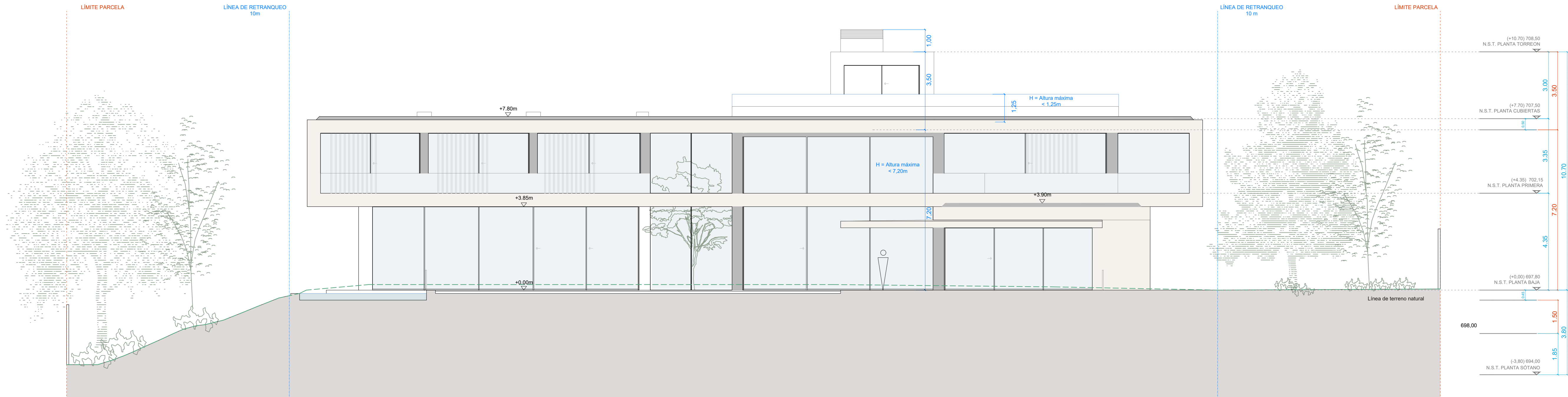
ALZADO SUR
