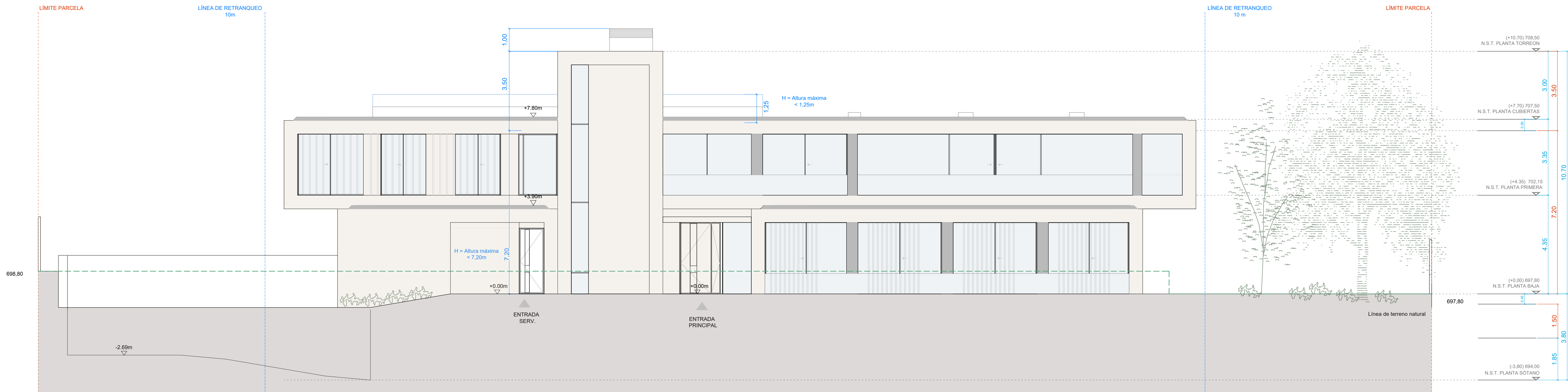
ALZADO NORTE
