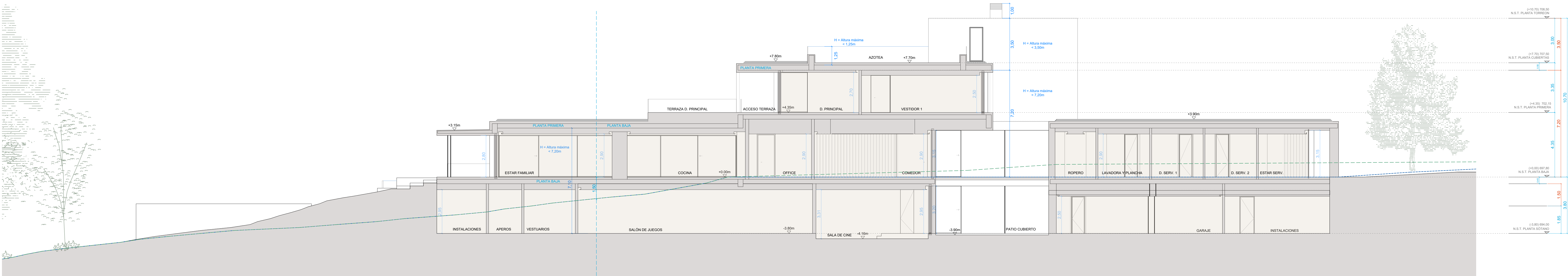
SECCIÓN A-A'
