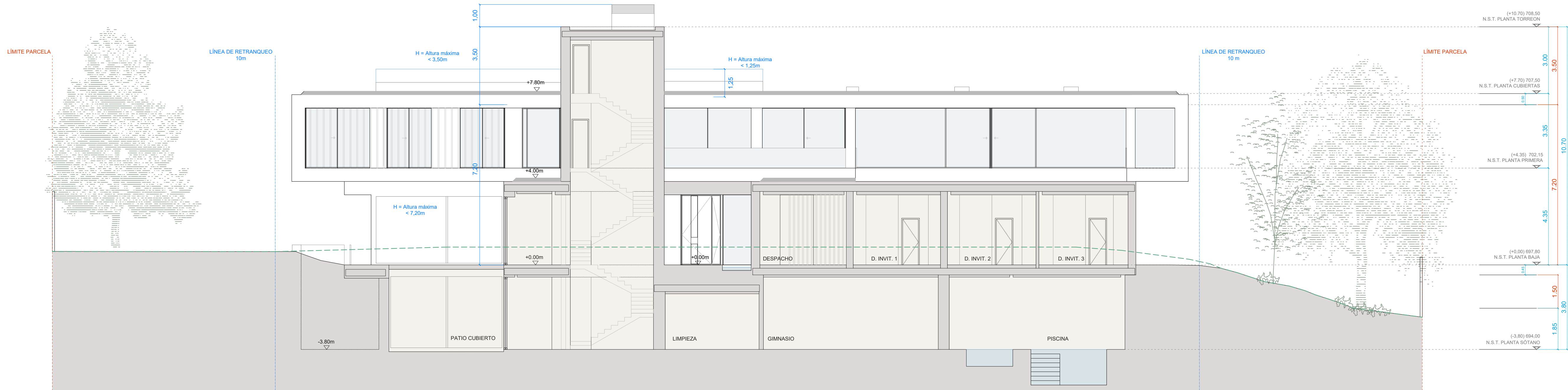
SECCIÓN G-G'
