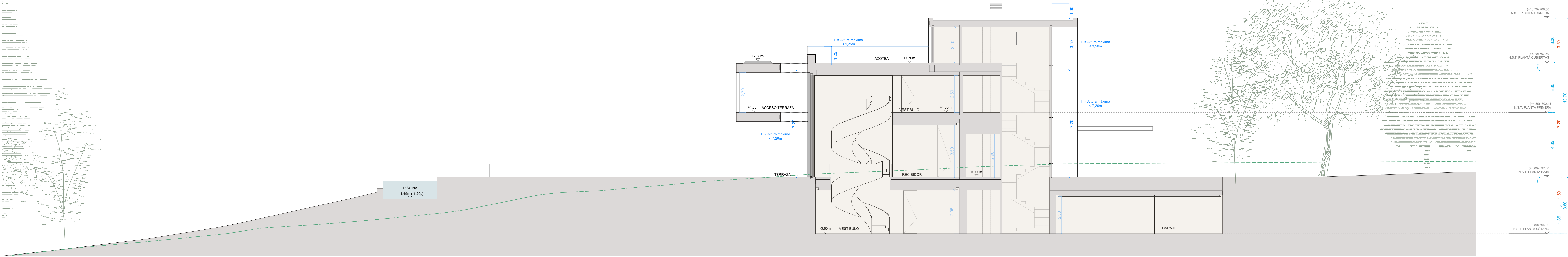
SECCIÓN B-B'
