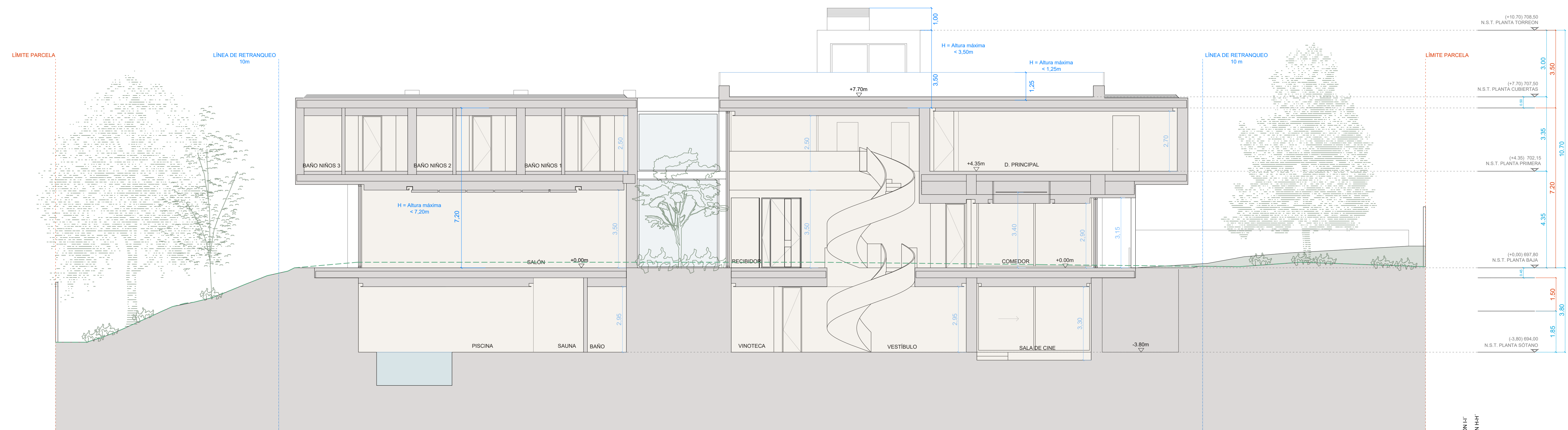
SECCIÓN H-H'
