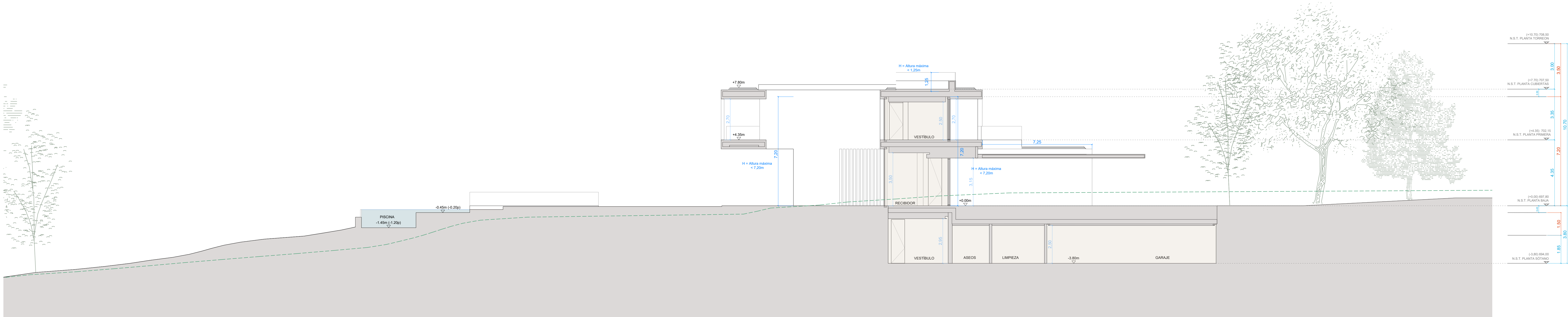
SECCIÓN C-C'
