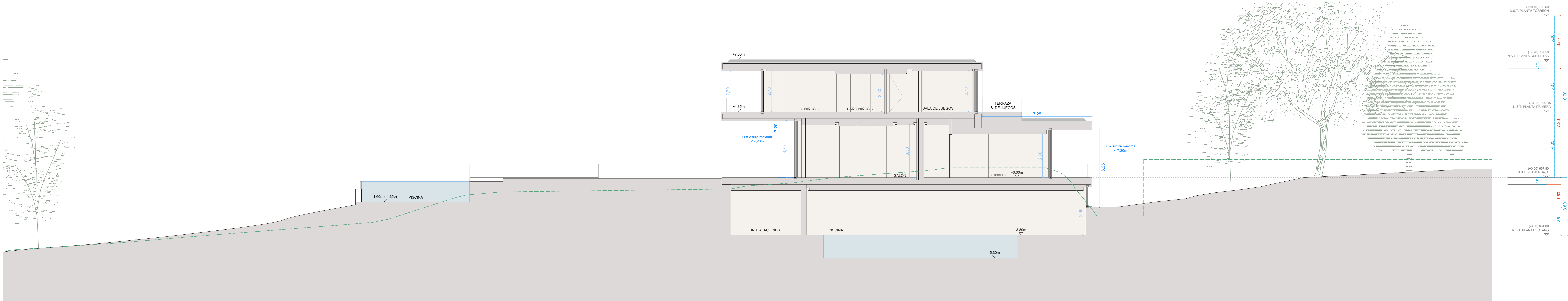
SECCIÓN D-D'
