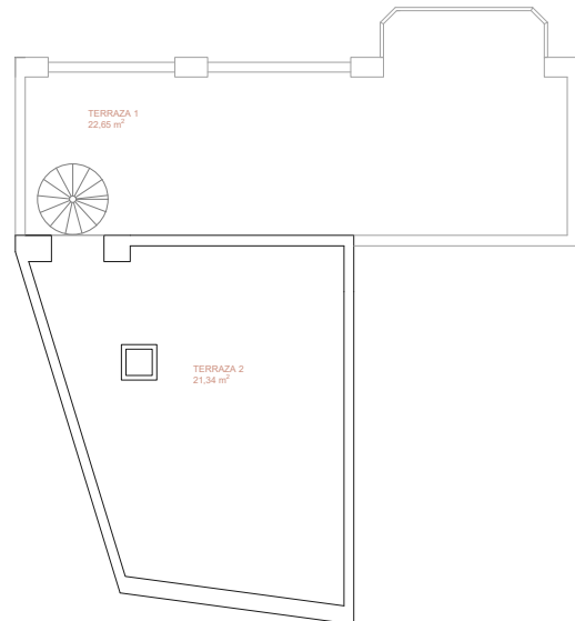
PLANTA SEGUNDA
