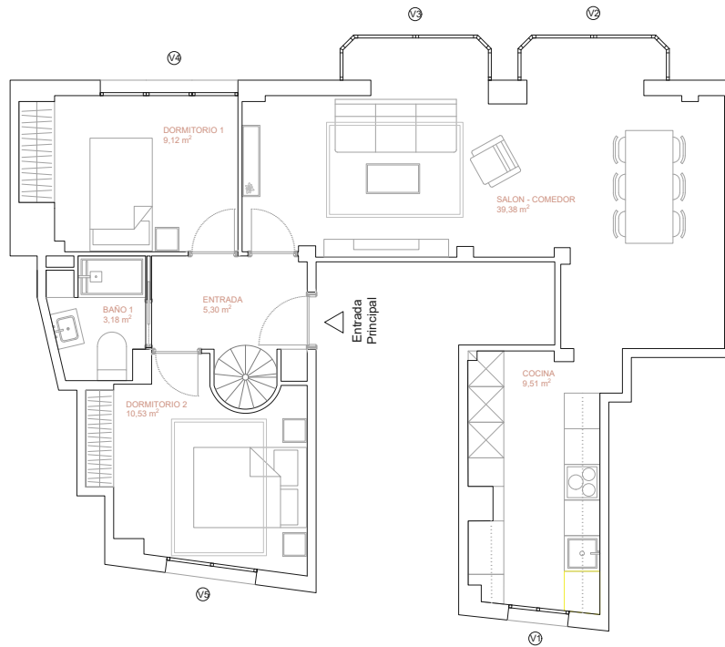
PLANTA BAJA
