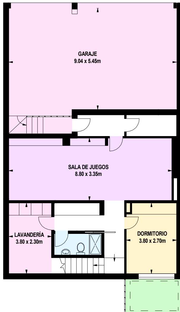
PLANTA SÓTANO
