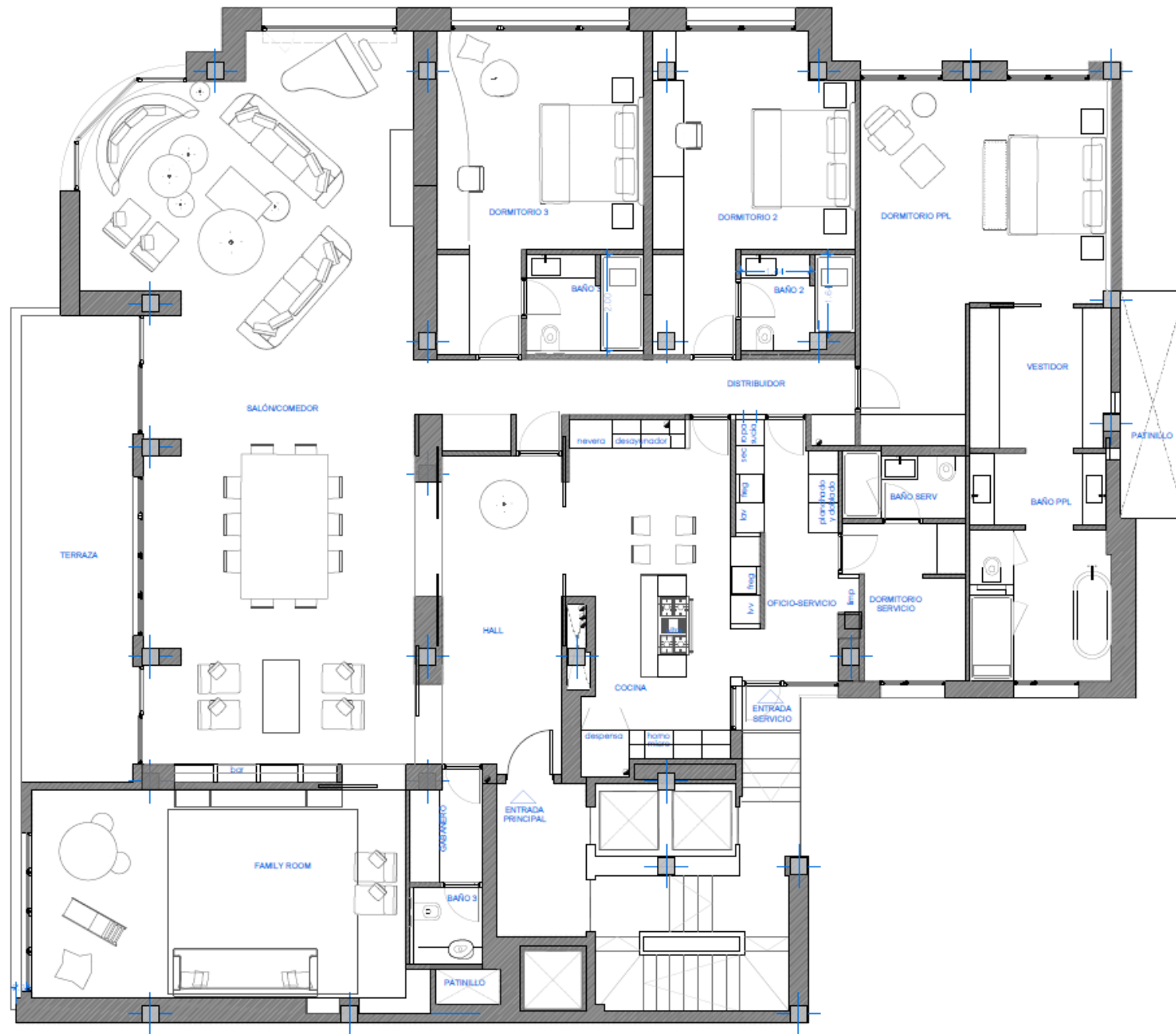
PLANTA 3º
