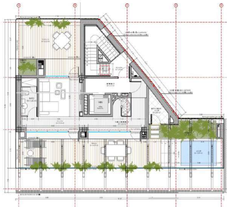
PLANTA NIVEL 06_COTA +22.00m
