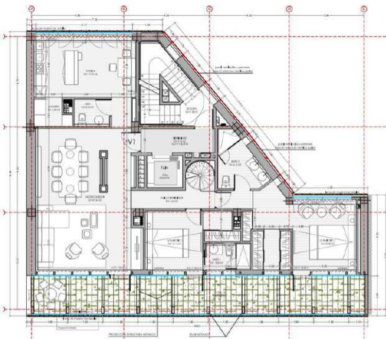
PLANTA NIVEL 05_COTA +18.00m
