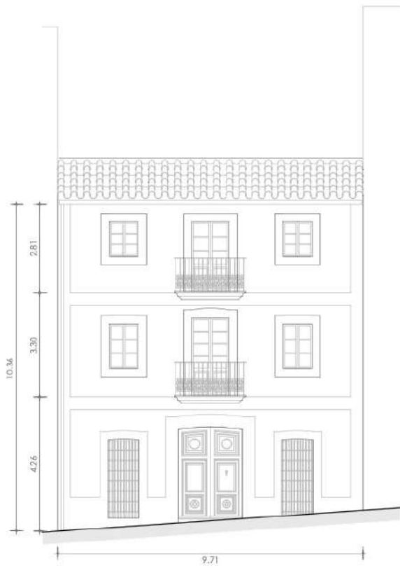
Fachada Anterior
