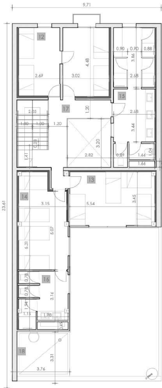
Planta Segunda
