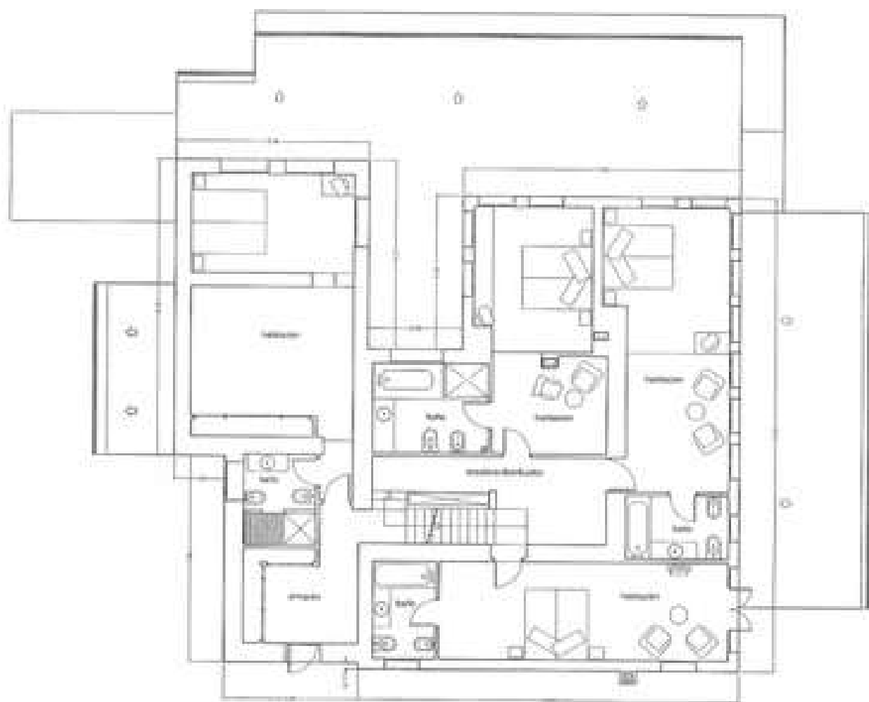
PLANTAS DE DISTRIBUCIÓN 3-Vivienda; Planta primera; 202,75 m 2
