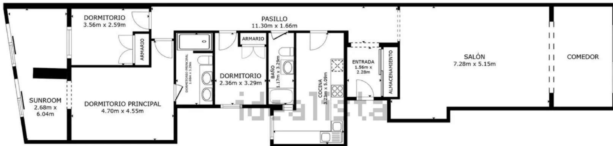
PLANTA
