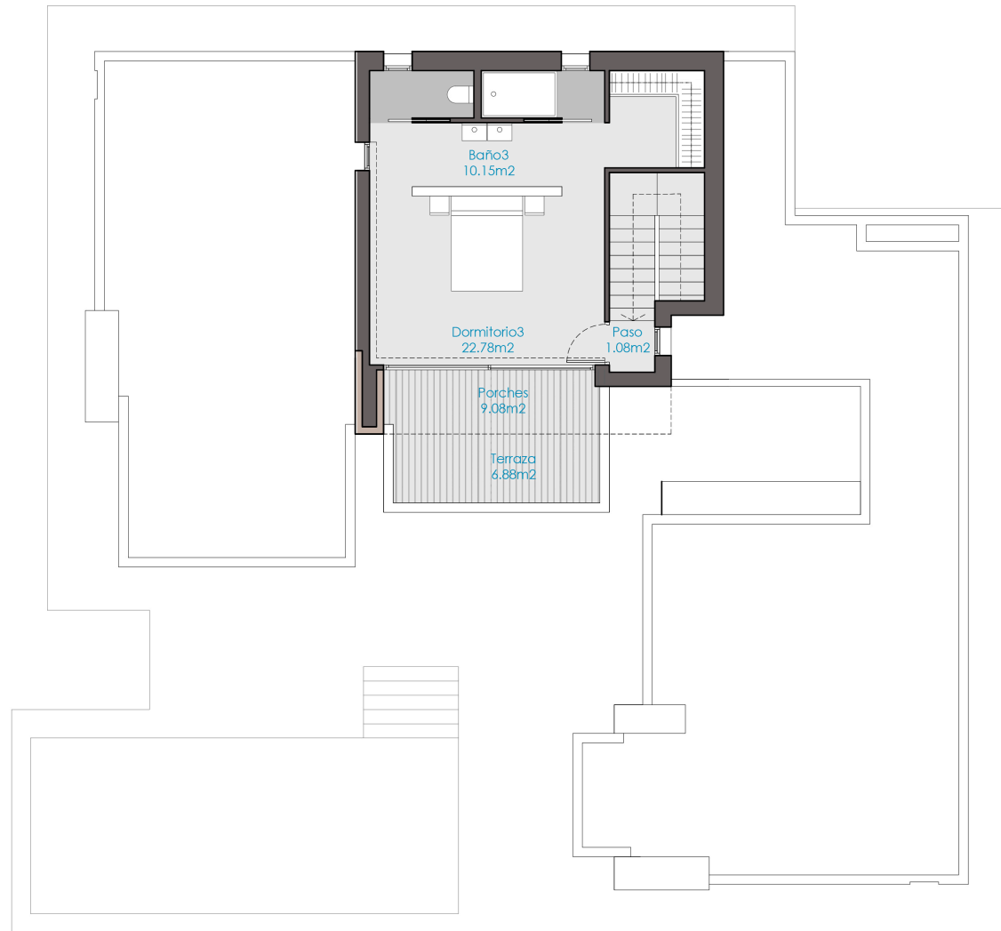
PLANTA ALTA
