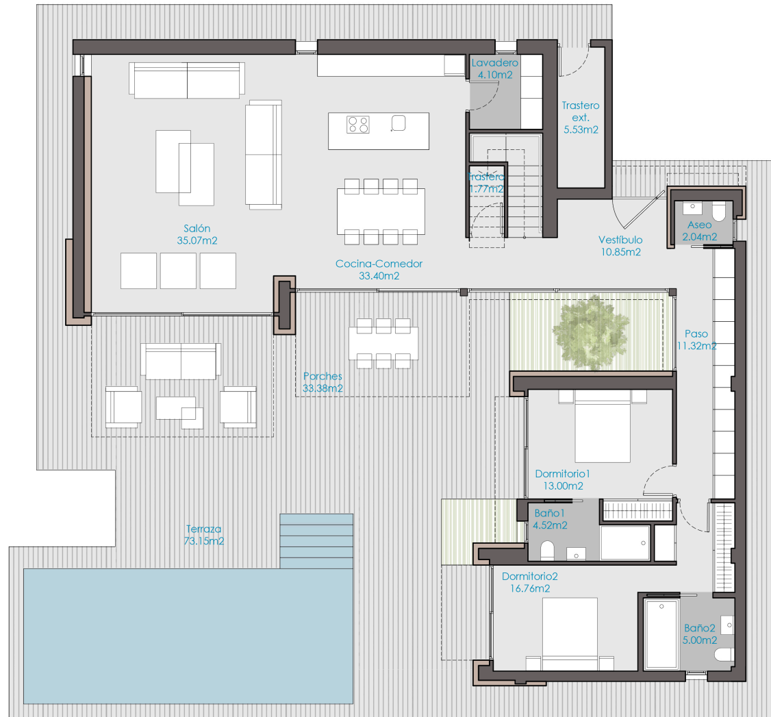
PLANTA BAJA
