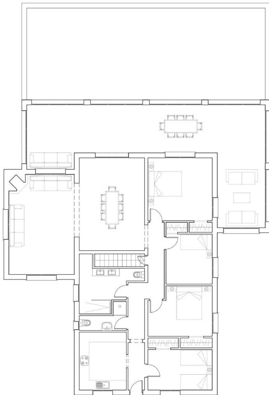
PLANTA BAJA
