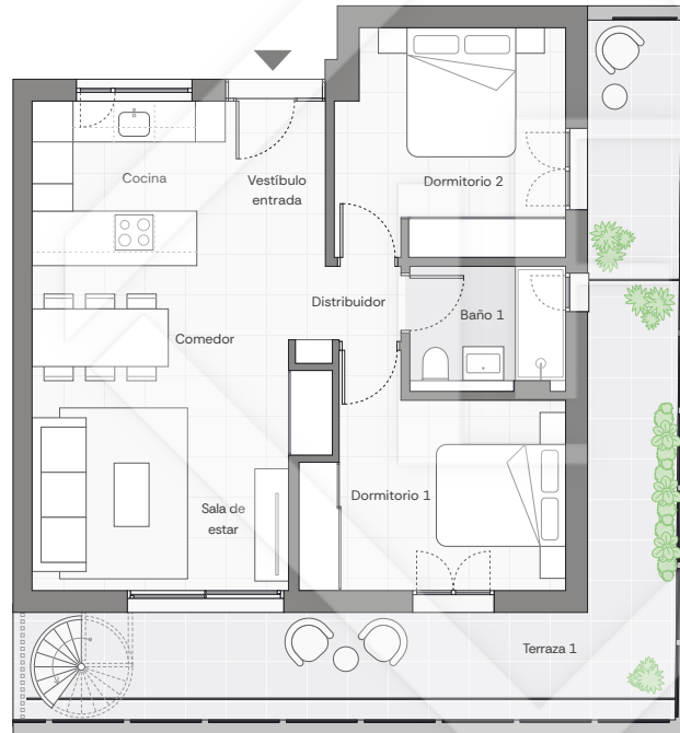
PLANTA VIVIENDA
