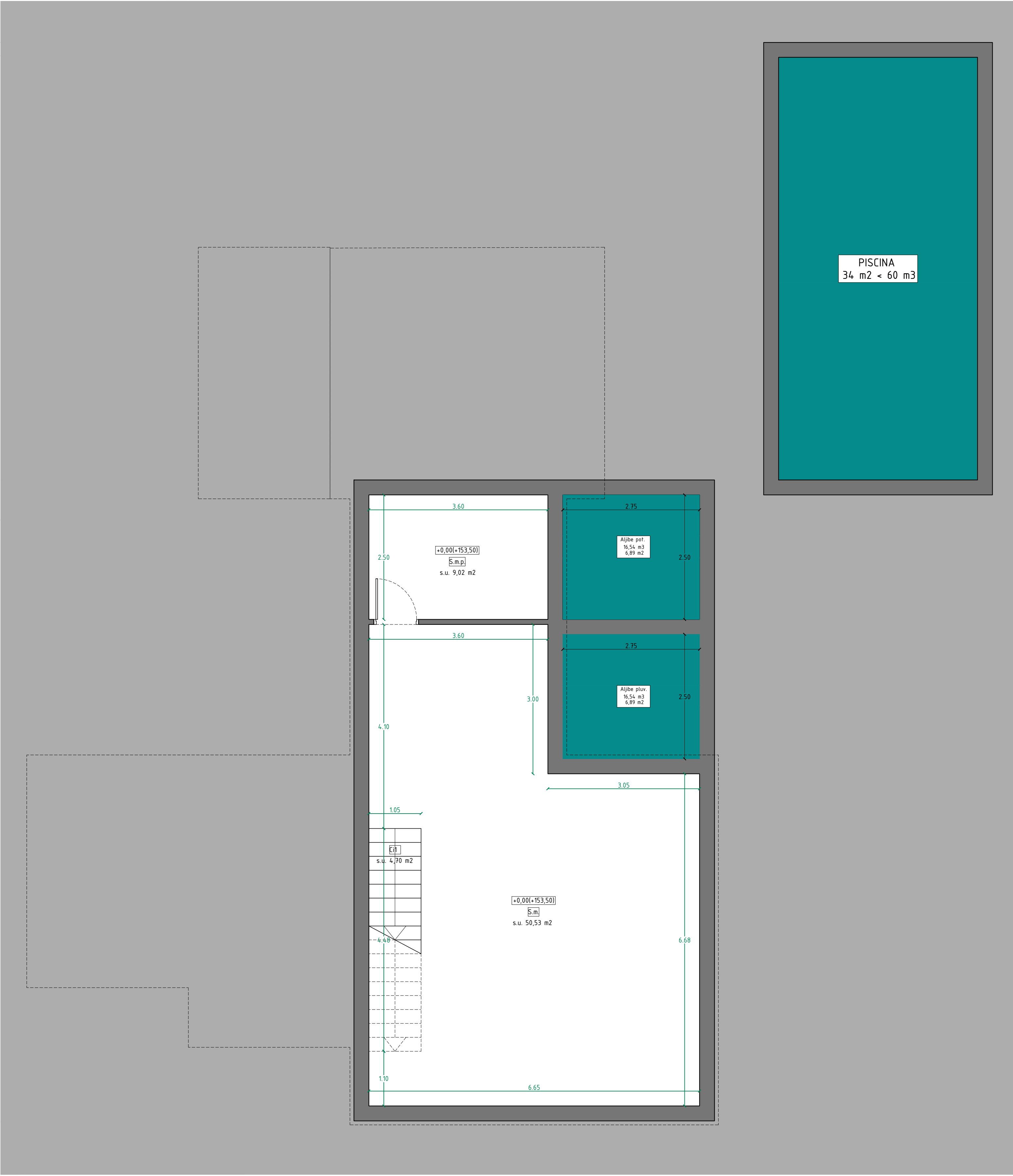
Pl. Cotas planta sótano e 1'50
