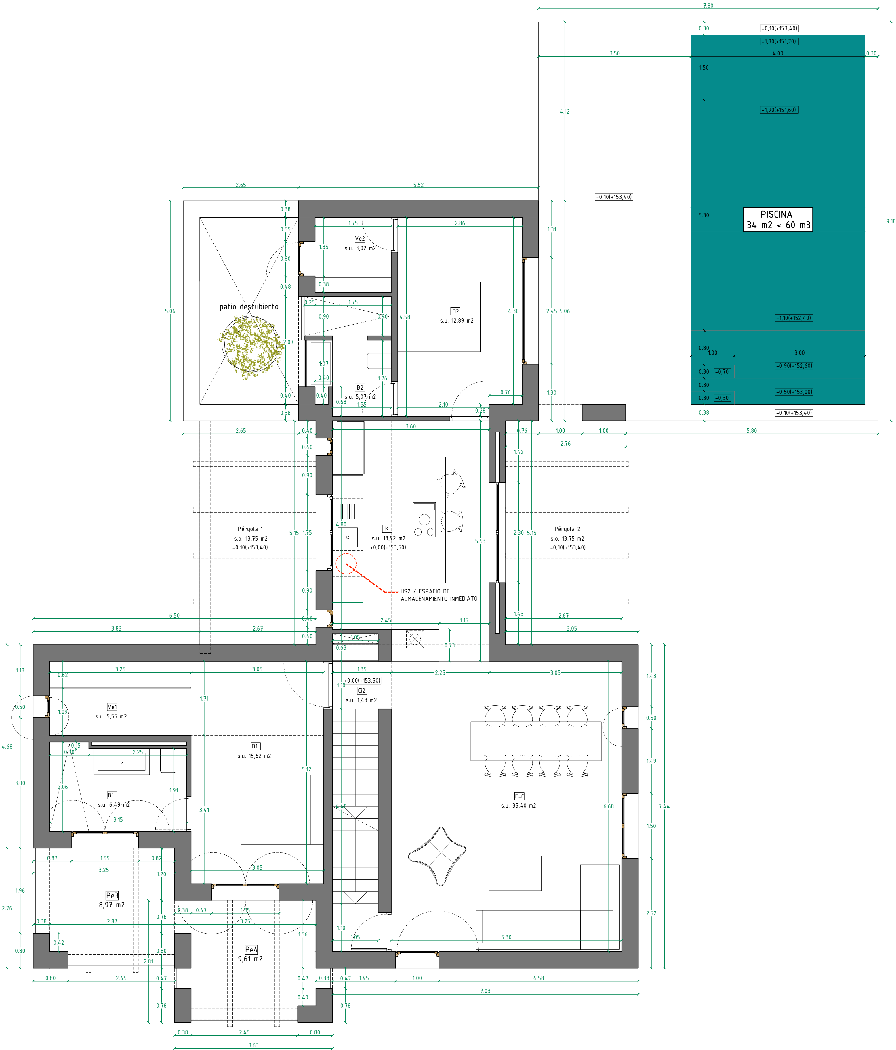
Pl. Cotas planta baja e 150
