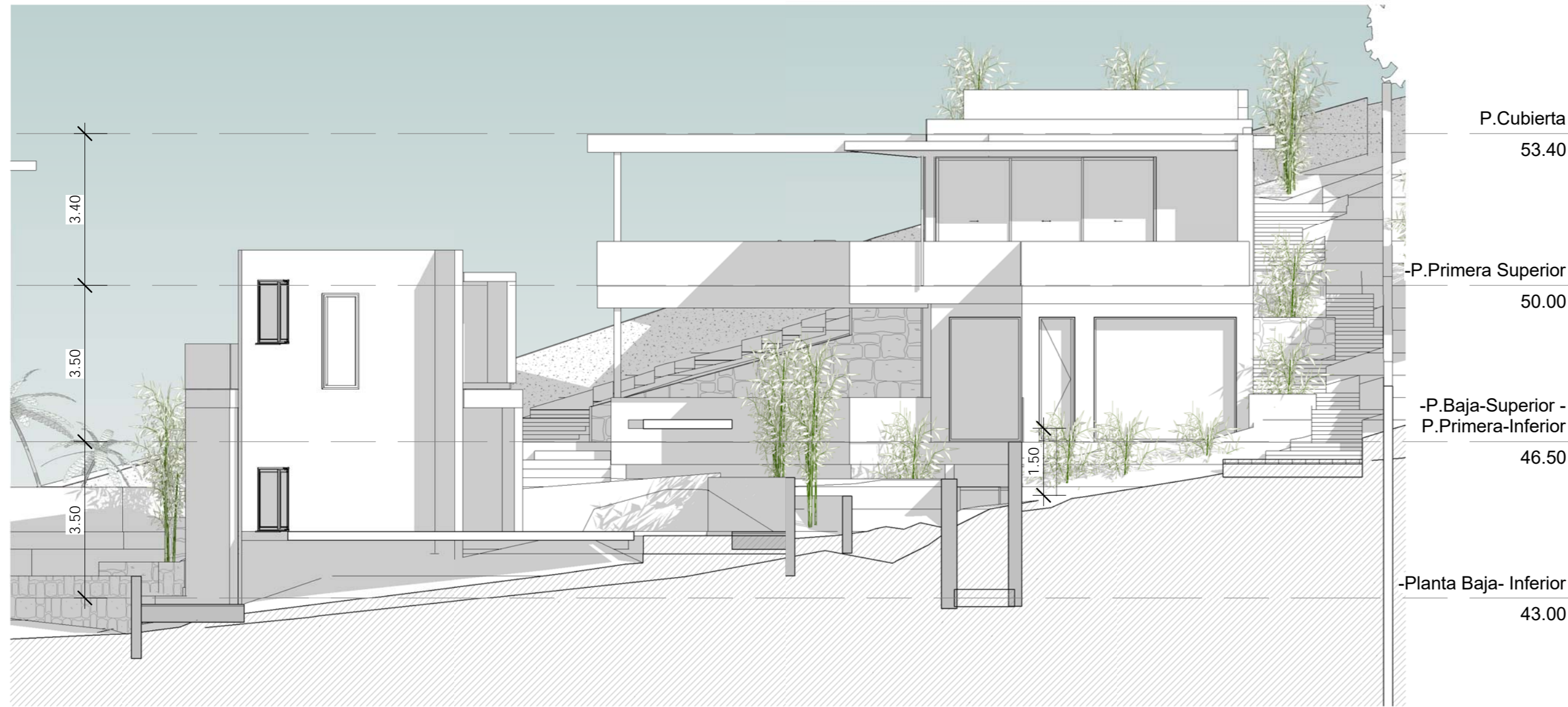
ALZADO SUR
