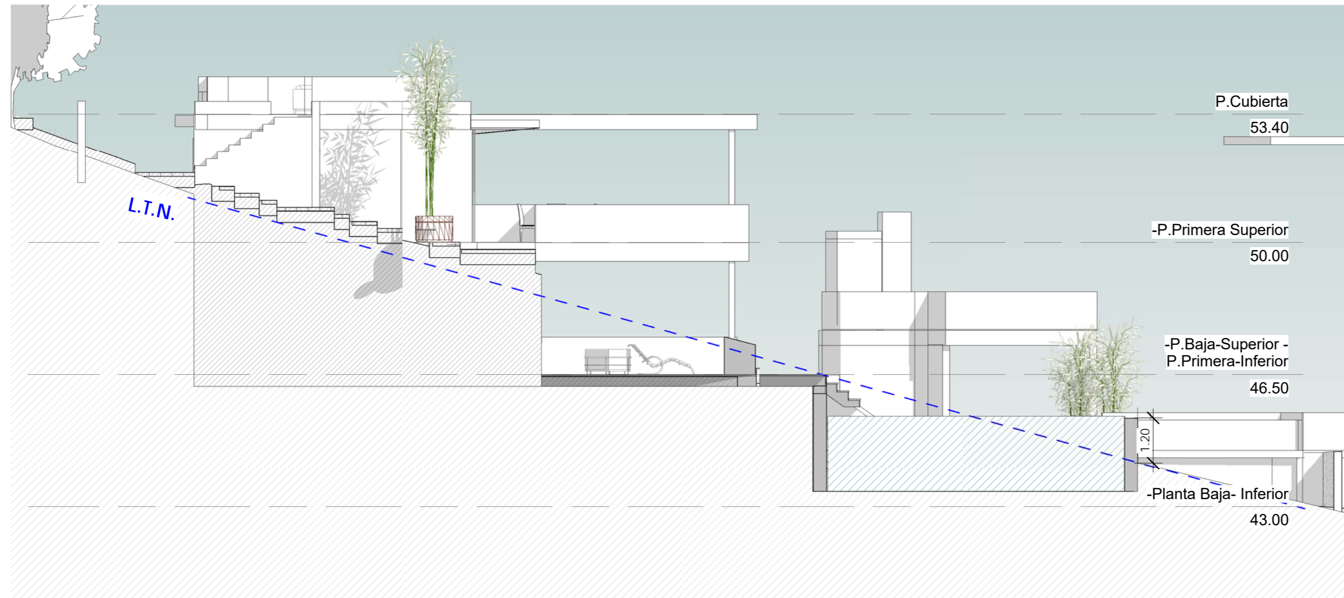
ALZADO NORTE
