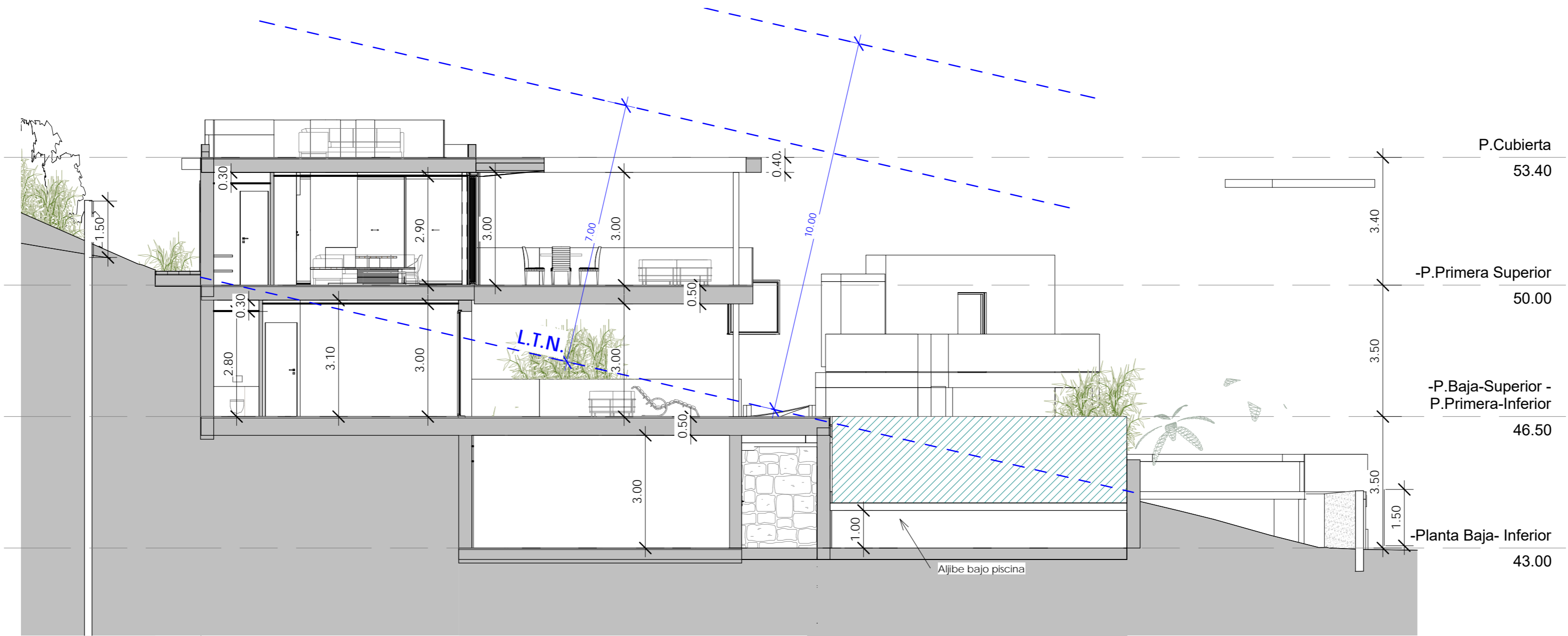
SECCIÓN 1
