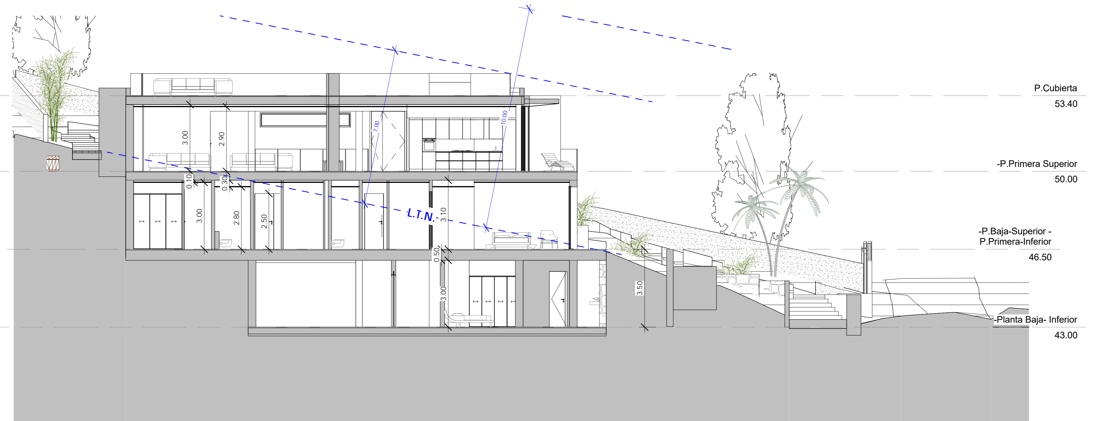
SECCIÓN 2
