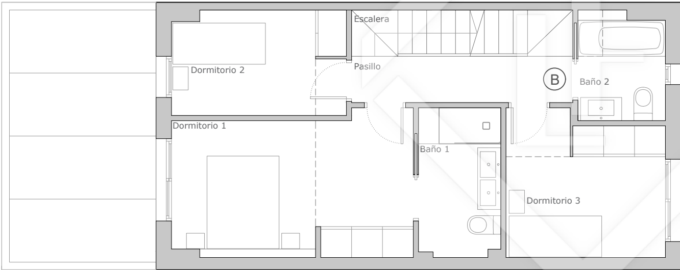
PLANTA SEGUNDA
