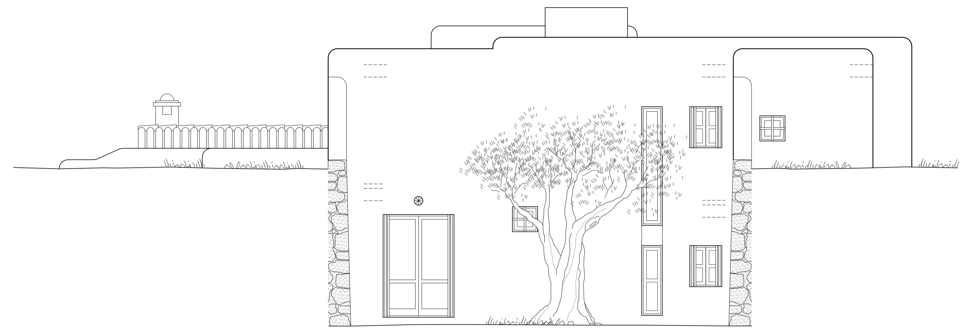
ALZADO OESTE.
