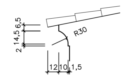
DETALLE ALERO TEJA.
