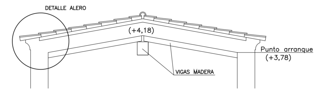
DETALLE CUBIERTA SALON FORJADO INCLINADO CON 18% DE PENDIENTE CON VIGAS FALSAS DE MADERA POR DEBAJO
