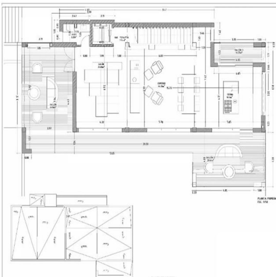
PLANTA DE COBERTA ESC. 1/50
