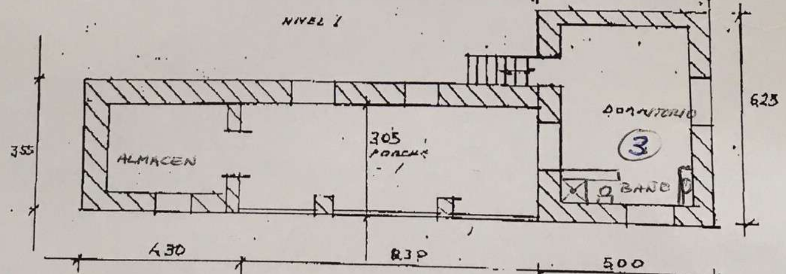
PLANTA PISO
