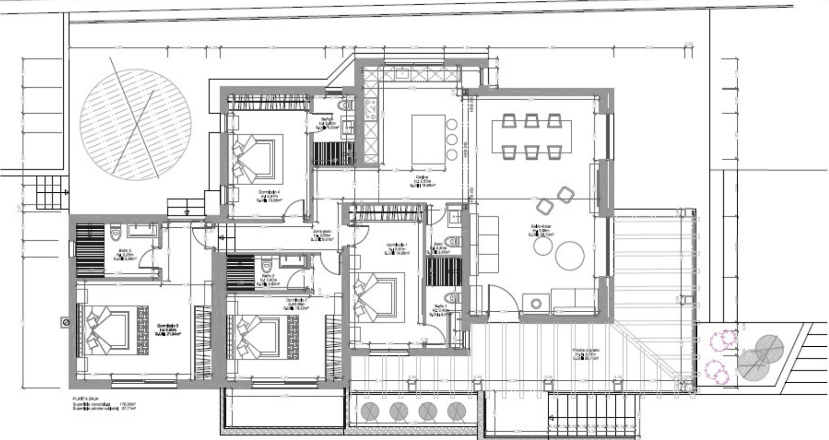
Planta Cubierta E-1/250
