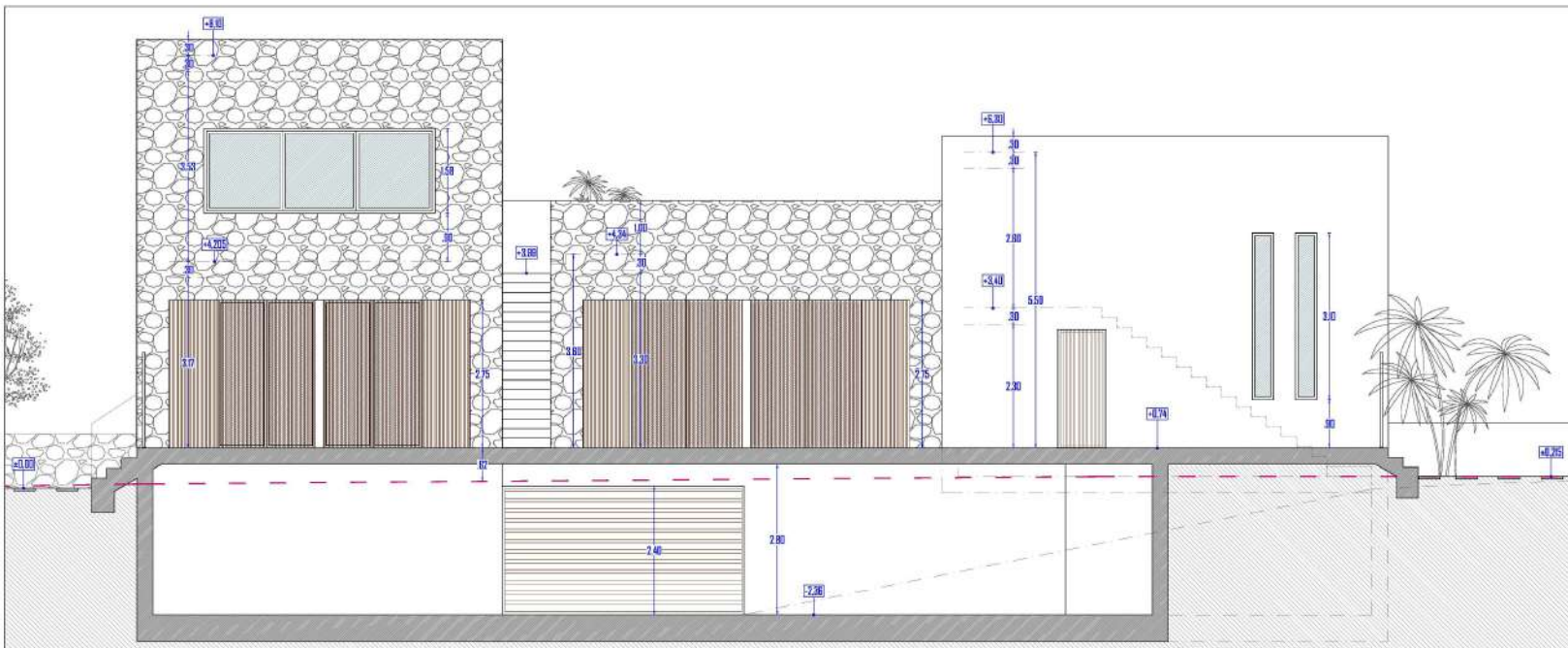
ALZADO ESTE - INTERIOR PATIO
