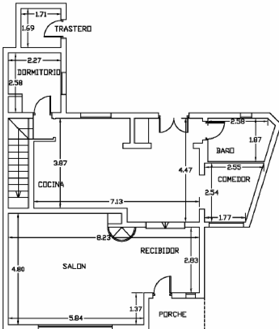
PLANTA BAJA
