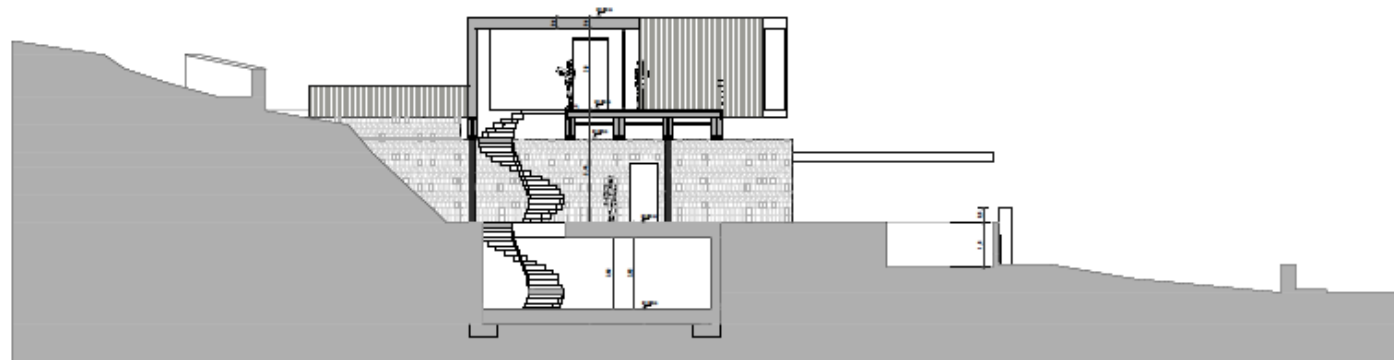
S 5_SECCIÓN TRANSVERSAL
