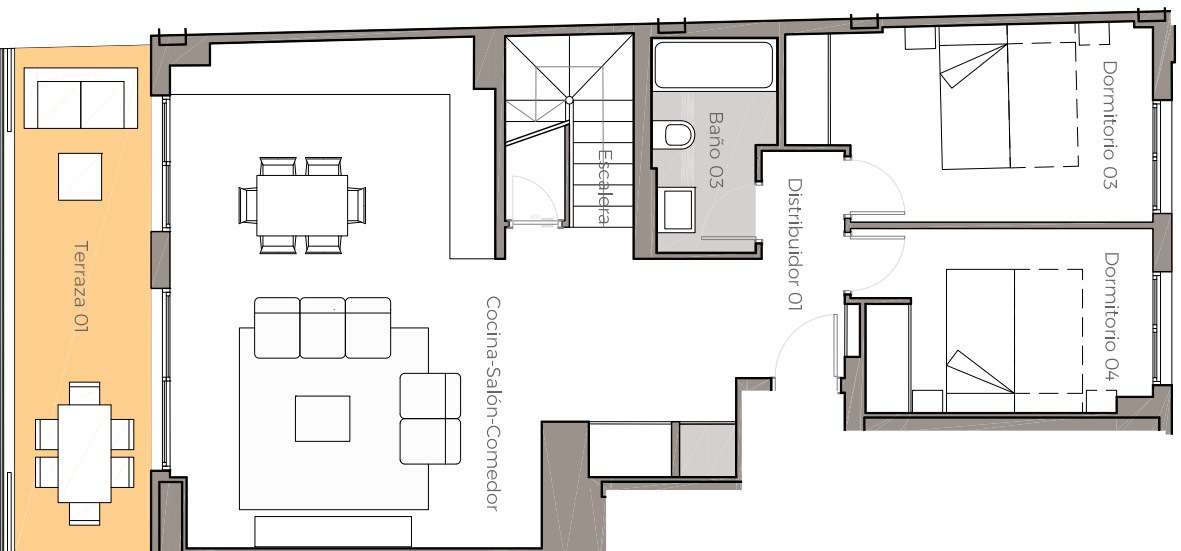
PLANTA TERCERA
