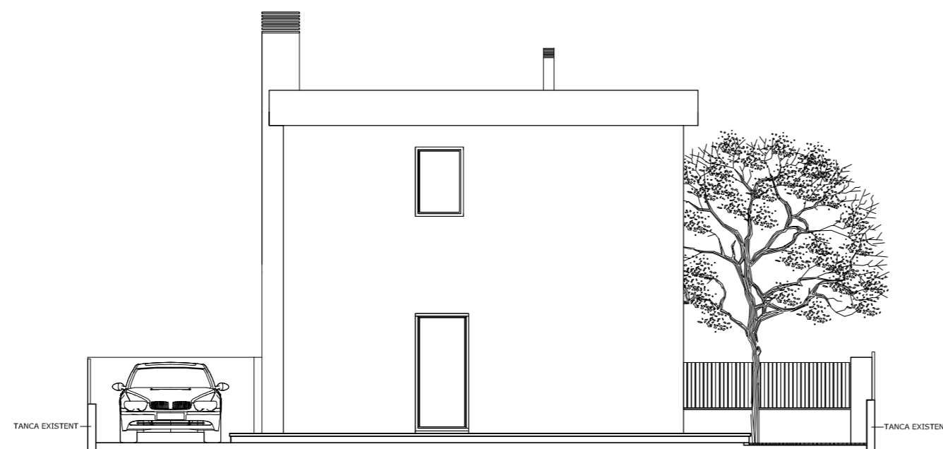
FAÇANA NORD
