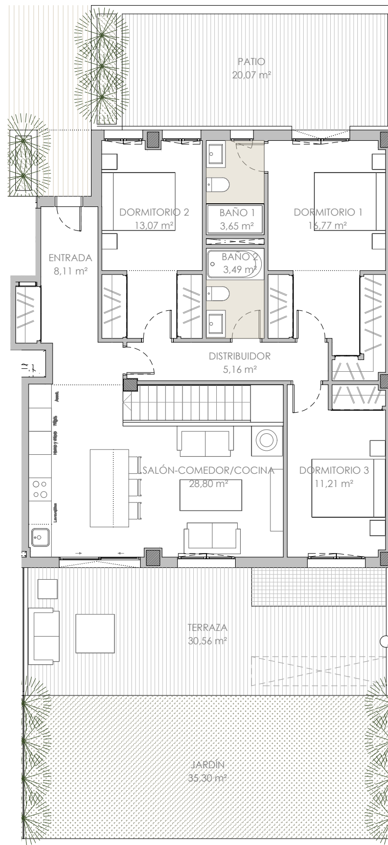
PLANTA BAJA
