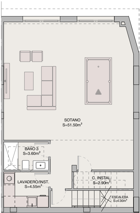
planta sotano
