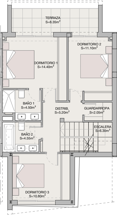
planta primera
