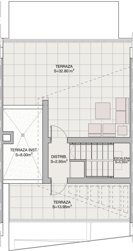
planta solarium
