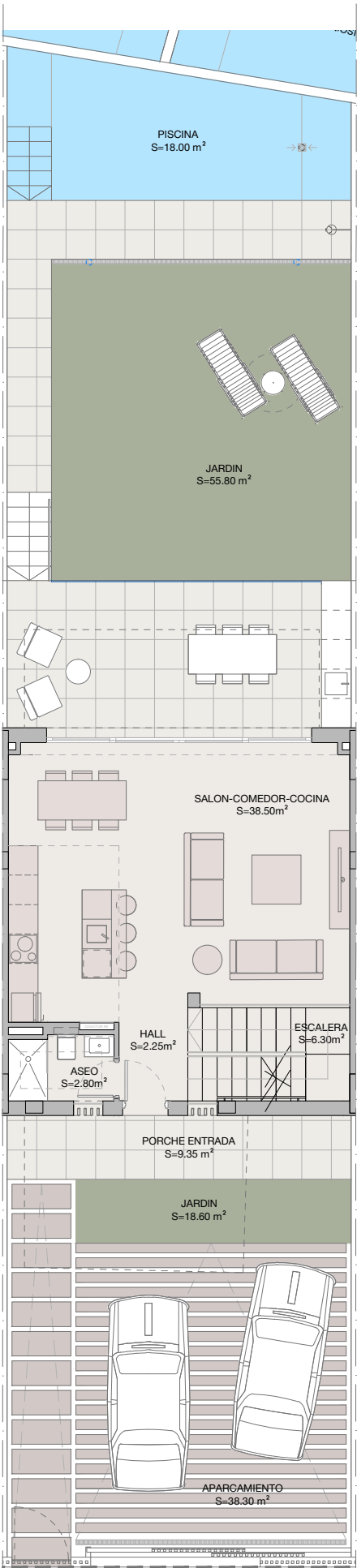
planta baja
