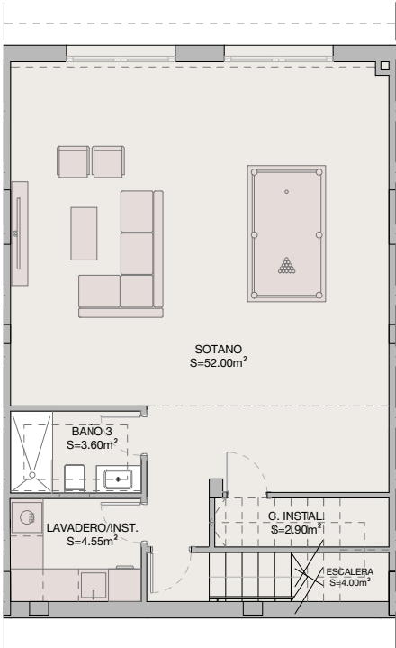
planta sotano
