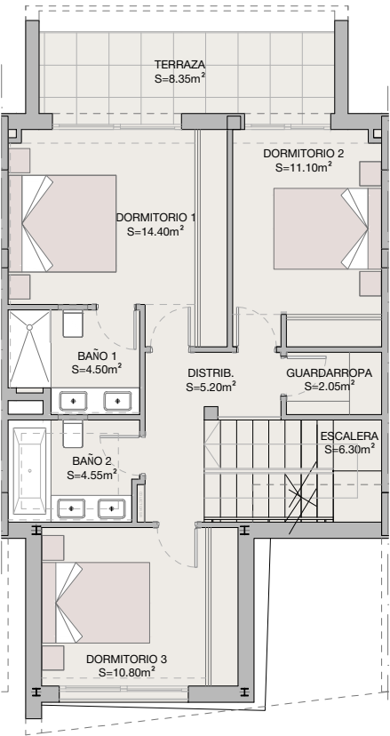
planta primera
