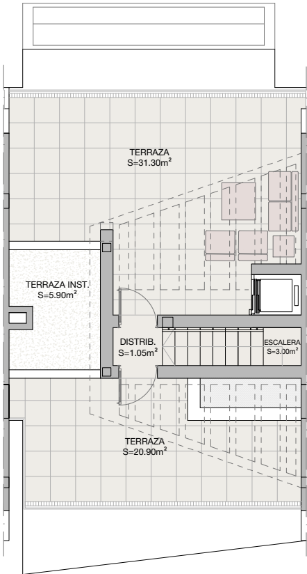
planta solarium
