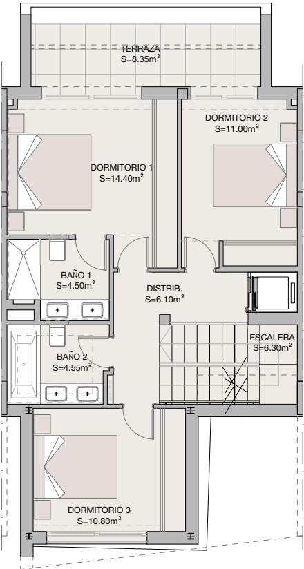
planta primera
