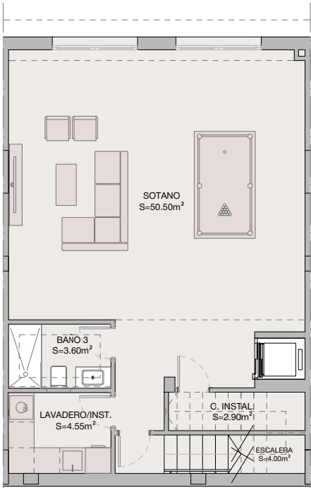
planta sotano
