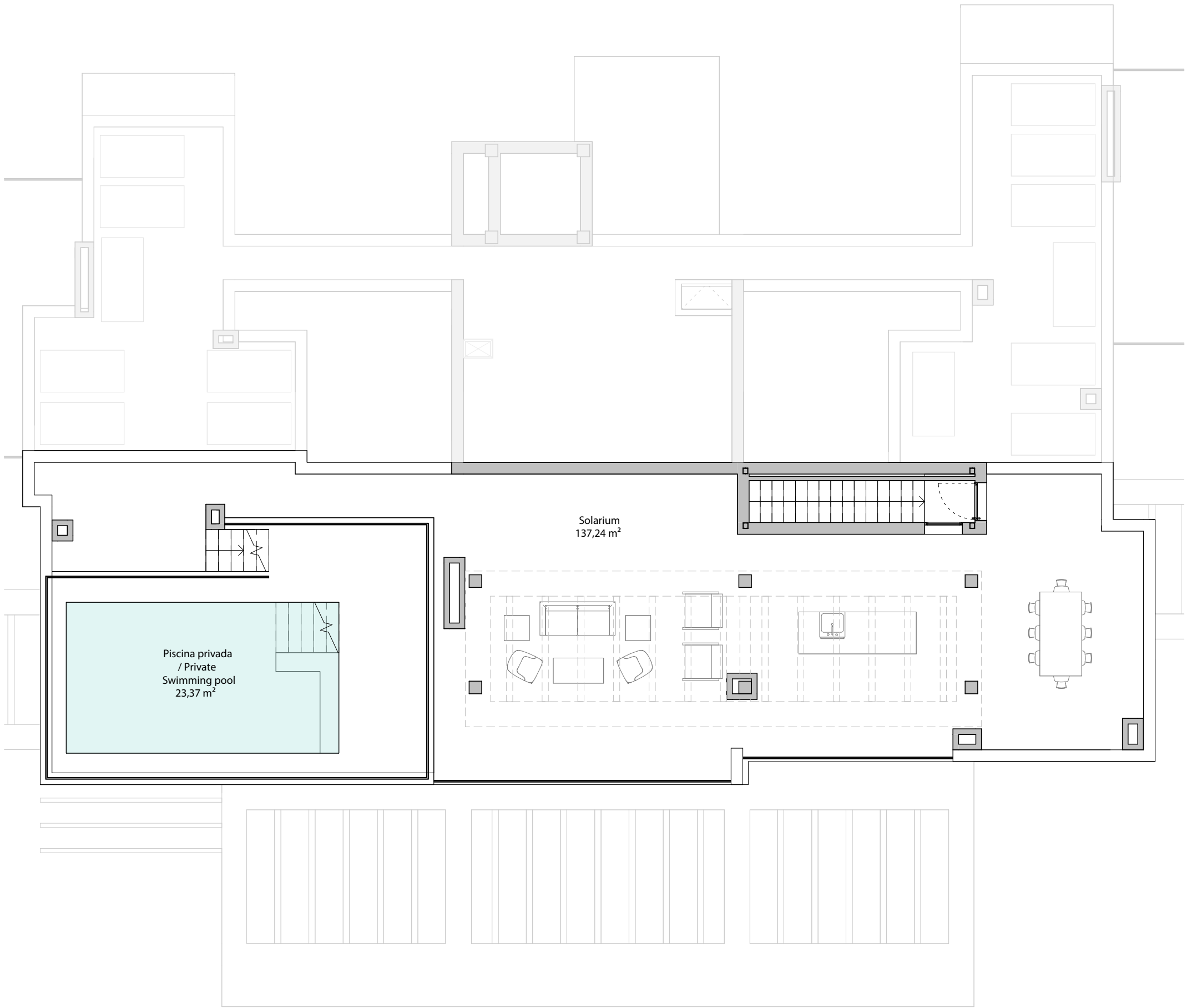
PLANTA SOLARIUM
