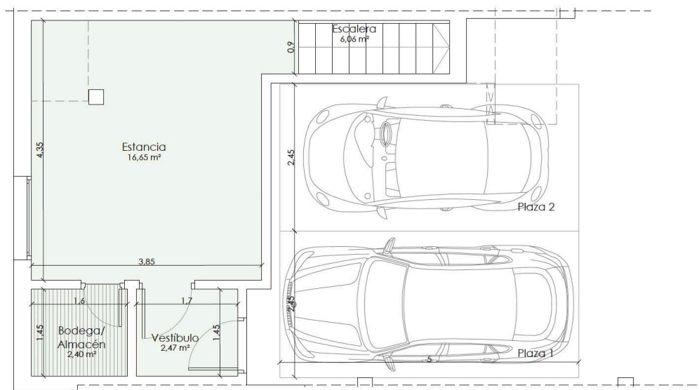
Garage/Basement
