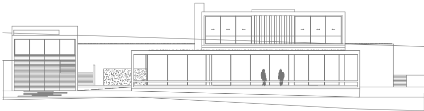
Alzado Oeste/West Elevation
